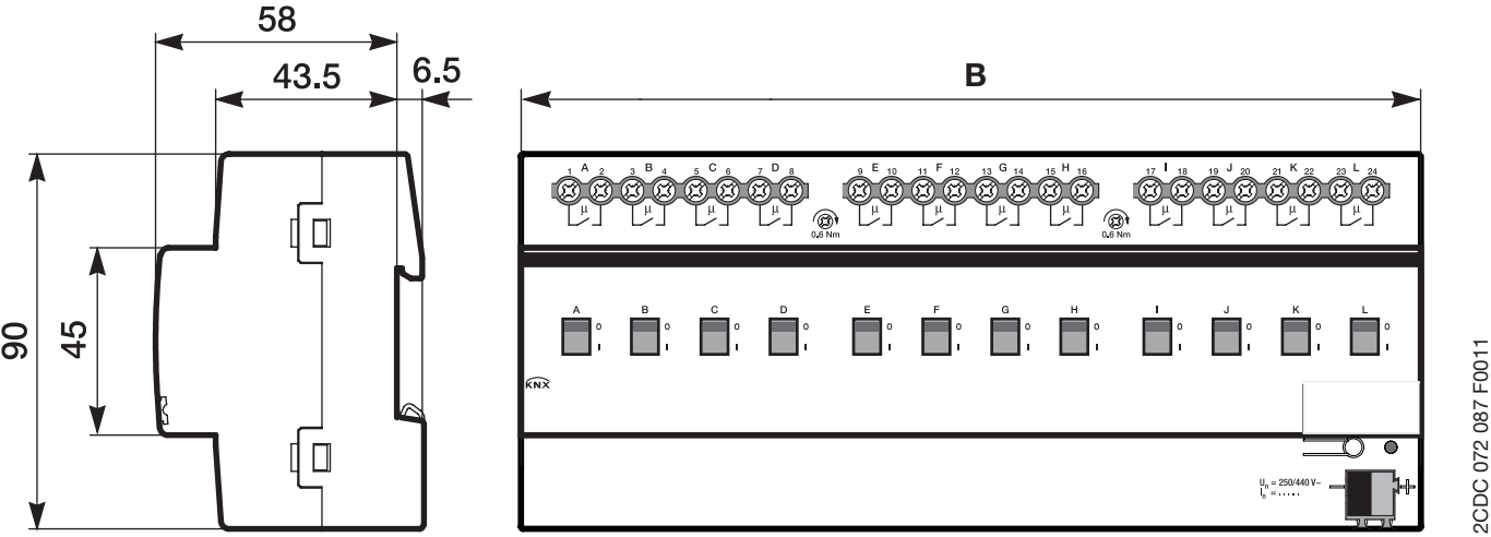
Maßbild SA/S x.16.2.1
