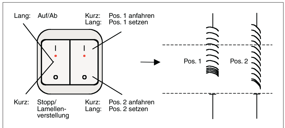
Abb. 5: Fahren in Preset-Position und Preset-Position speichern
