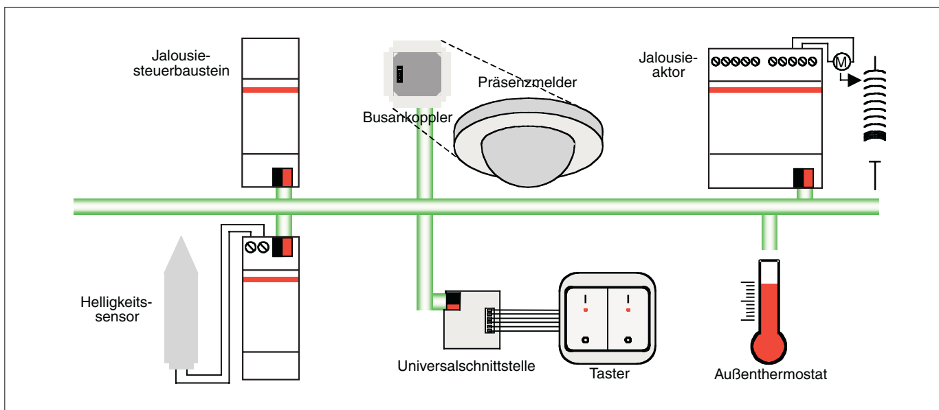
Abb. 14: Planung einer Heizen/Kühlen-Automatik-Steuerung
