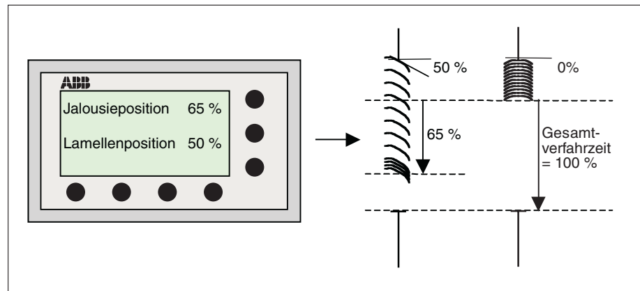
Abb. 4: Fahren in Position 0...100 %
