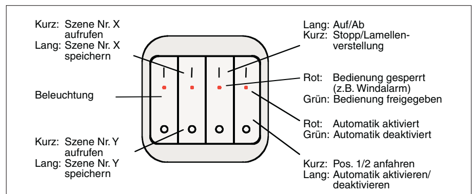
Abb. 17: Tasterbelegung Auf/Ab, Position anfahren, Automatik
