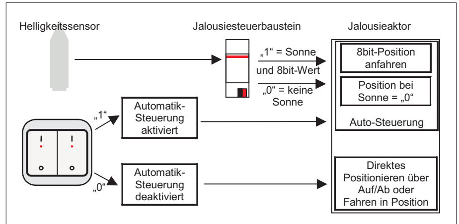
Abb. 10: Aufbau einer Sonnenschutz-Automatik-Steuerung mit Sonnenstandsnachführung
