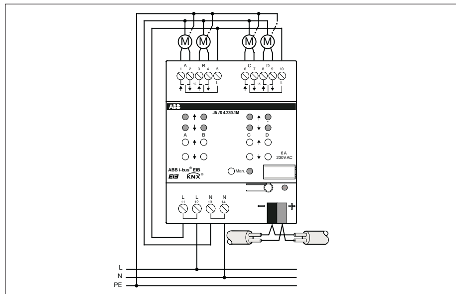
Abb. 15: Planung einer Spannungsüberwachung in den Schaltkreisen
