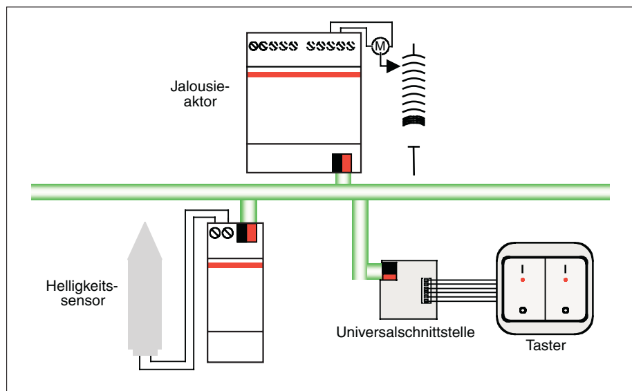
Abb. 9: Planung einer einfachen Sonnenschutz-Automatik-Steuerung
