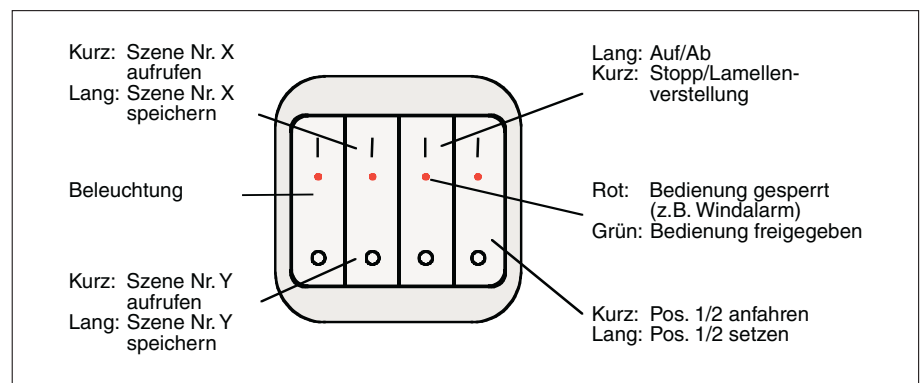
Abb. 16: Tasterbelegung Auf/Ab, Position anfahren, Position setzen
