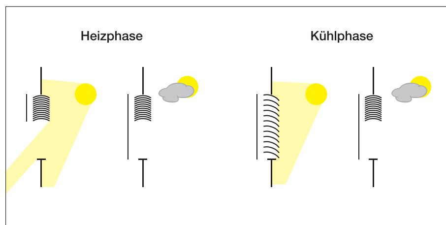
Abb. 12: Funktionsweise einer Heizen/Kühlen-Automatik-Steuerung
