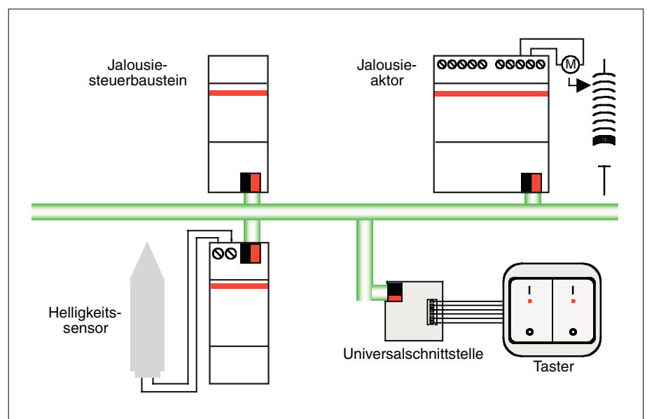
Abb. 11: Planung einer Sonnenschutz-Automatik-Steuerung mit Sonnenstandsnachführung
