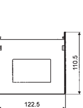
Abdeckung lang
