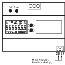
M-Bus
