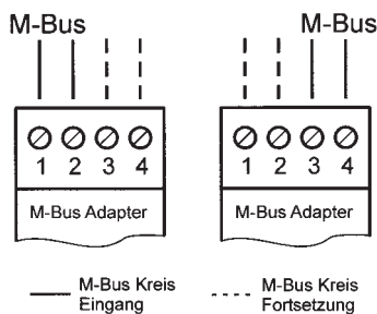
Bild 3: Anschluss Zwei-Leiter M-Bus
