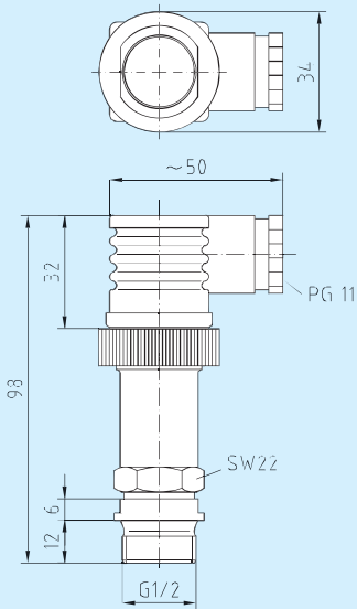
Maßzeichnung
