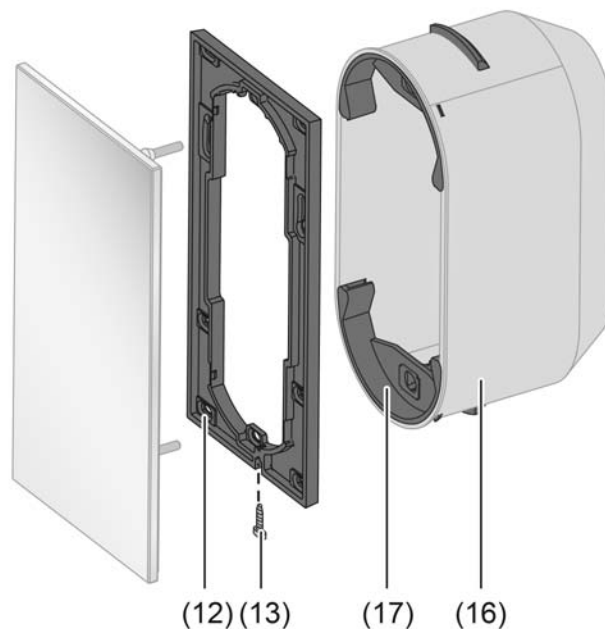
Bild 5: Gerätemontage eines Glas-Sensors TS Komfort mit erhöhtem Demontageschutz
