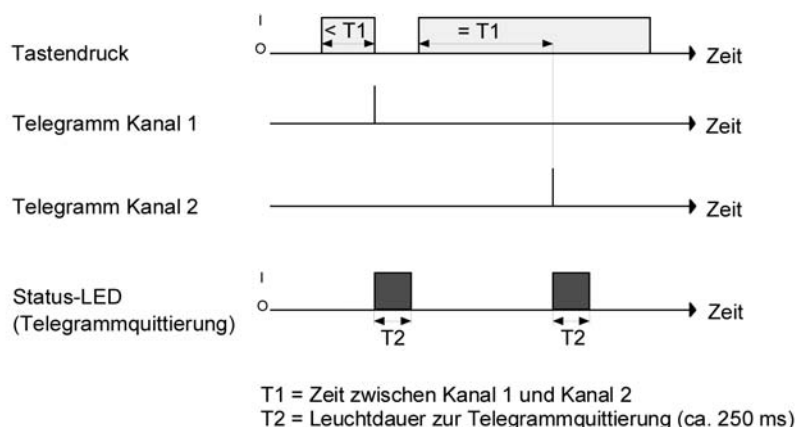
Bild 18: Beispiel zum Bedienkonzept "Kanal 1 oder Kanal 2"
