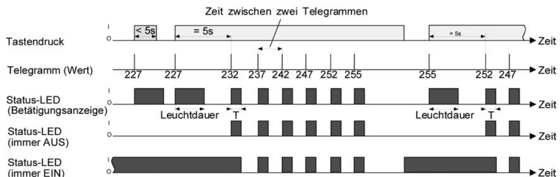
Bild 16: Beispiel zur Wertverstellung ohne Wertbereichs-Überlauf
