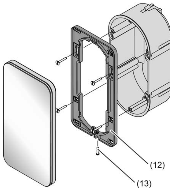
Bild 3: Gerätemontage eines Touch-Sensors Komfort
