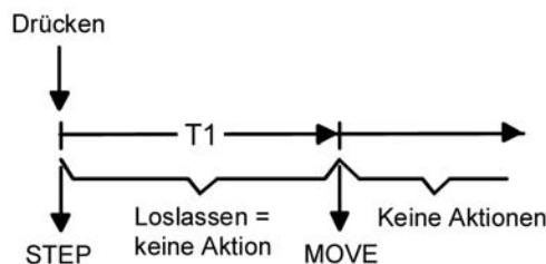
Bild 14: Bedienkonzept "Kurz - Lang"
