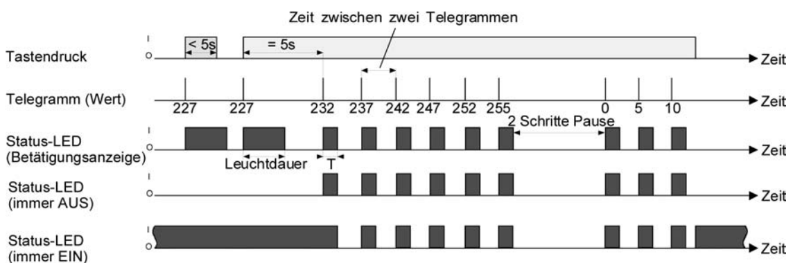
Bild 17: Beispiel zur Wertverstellung mit Wertbereichs-Überlauf
