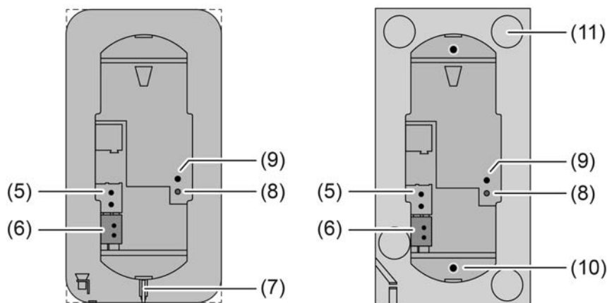
Bild 2: Geräteaufbau Rückseite links: R.x-Design / rechts: TS-Sensor-Design
