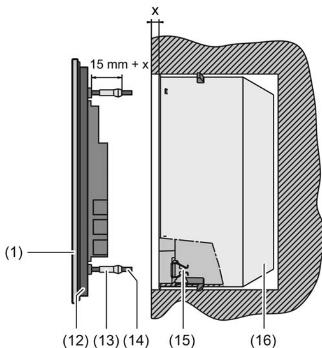
Bild 4: Gerätemontage eines Glas-Sensors TS Komfort
