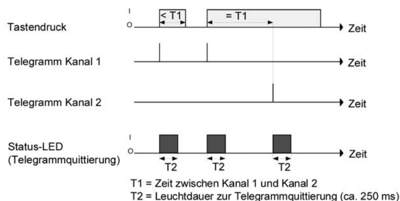
Bild 19: Beispiel zum Bedienkonzept "Kanal 1 oder Kanal 2"
