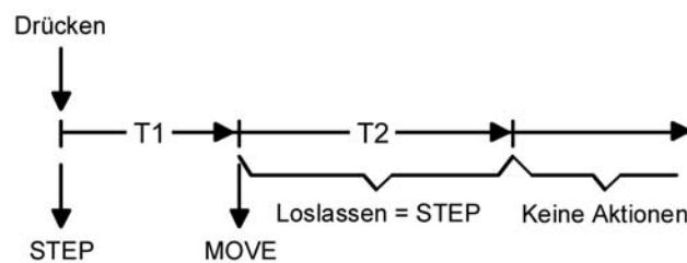
Bild 12: Bedienkonzept "Kurz-Lang-Kurz"
