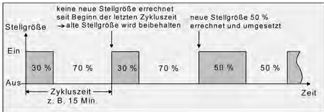
Bild 29: Schaltende PI-Regelung
