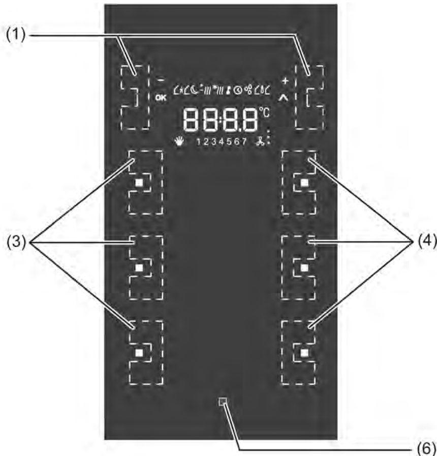
Bild 14: Tastenanordnung (am Beispiel der Gerätevariante 3fach)
