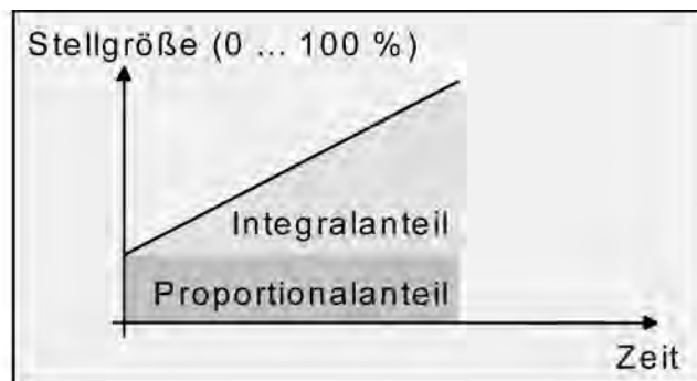
Bild 28: Stetige PI-Regelung
