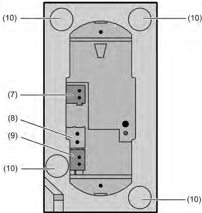
Bild 3: Geräteaufbau Rückseite
