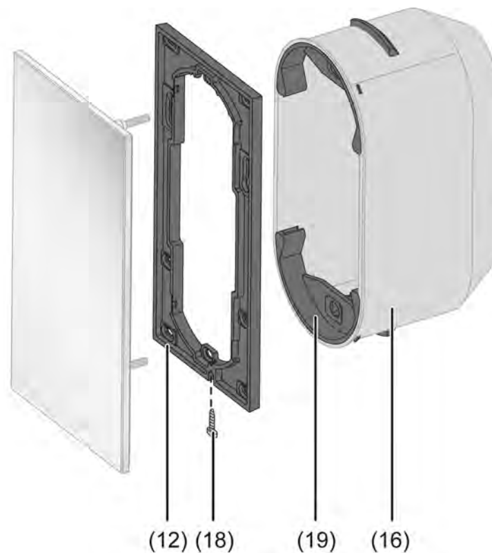
Bild 6: Befestigung auf Unterputz-Einbaudose mit erhöhtem Demontgaeschutz
