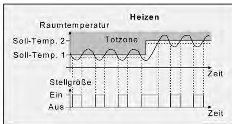
Bild 32: 2-Punkt-Regelung für Mischbetriebsart "Heizen und Kühlen" bei aktivem Heizbetrieb
