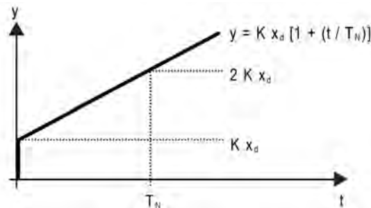
Bild 34: Funktion der Stellgröße einer PI-Regelung
