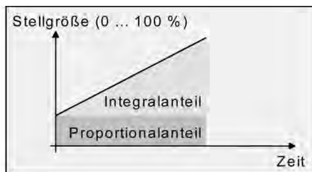
Bild 28: Stetige PI-Regelung
