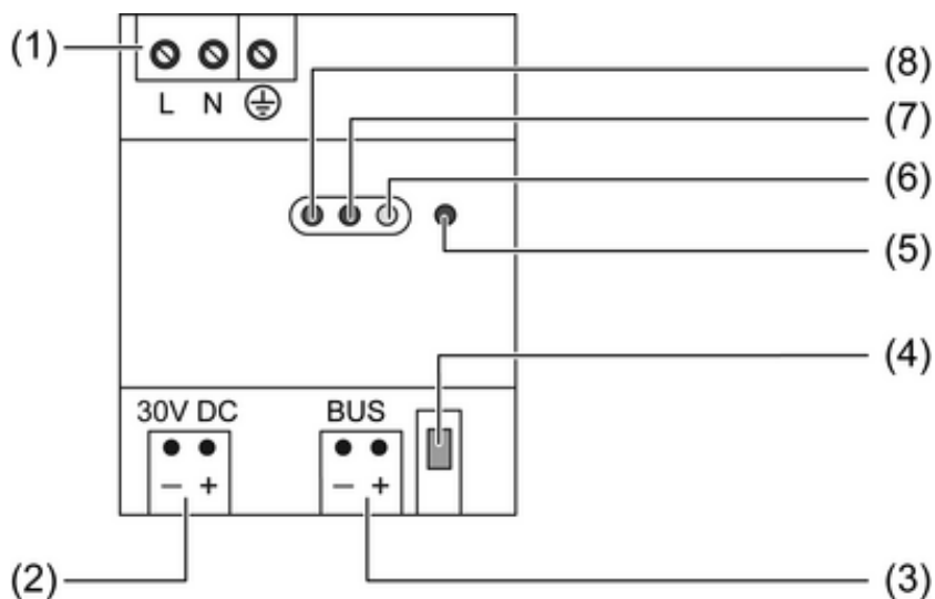
Bild 1: Spannungsversorgung 320 mA
