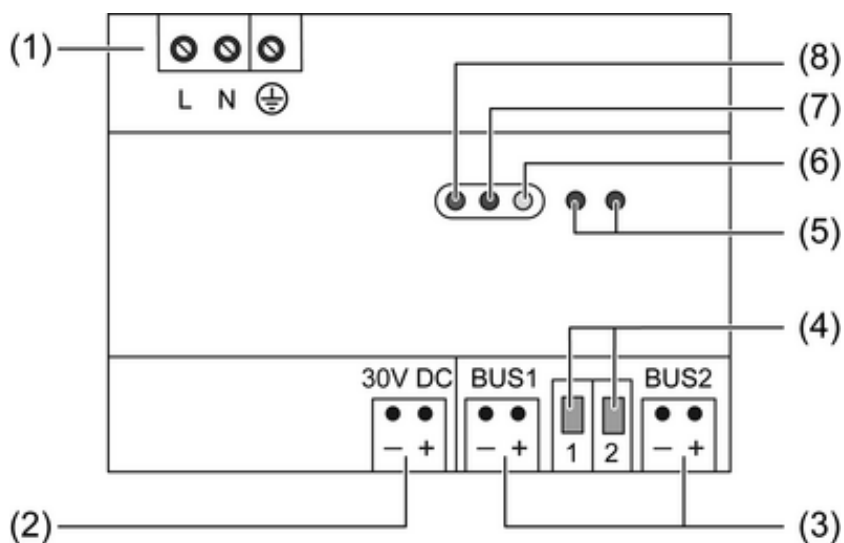
Bild 2: Spannungsversorgung 640 mA
