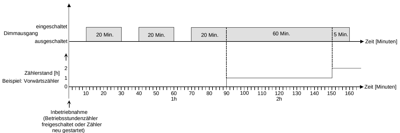
Bild 21: Funktionsweise des Betriebsstundenzählers
