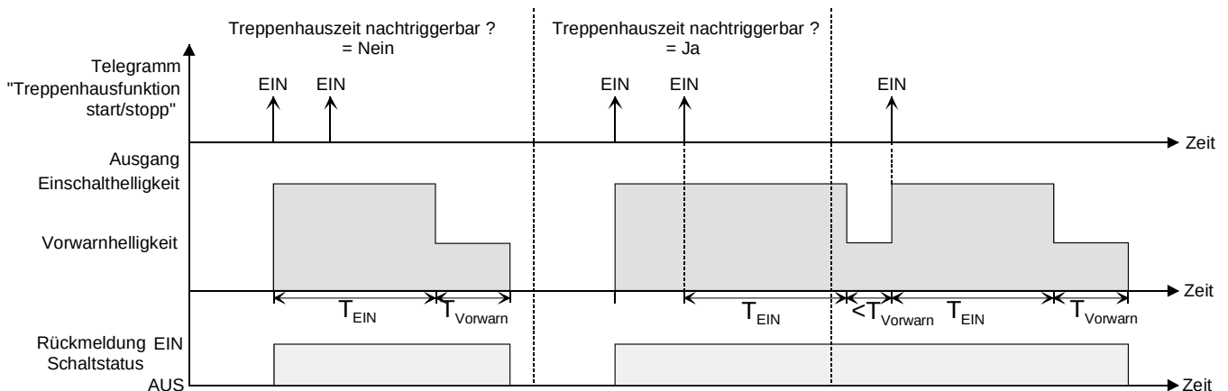
Bild 13: Einschaltverhalten der Treppenhausfunktion ohne Soft-Funktionen
