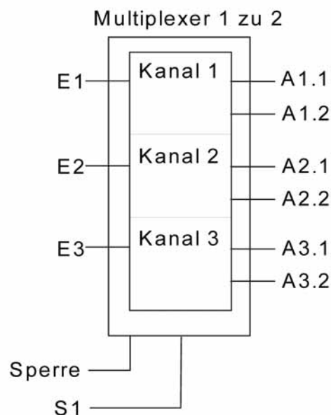
Bild 29: Multiplexer "1 zu 2"
