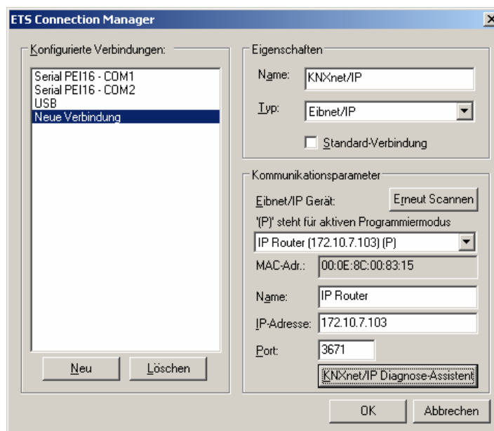
Bild 8: Vollständige Schnittstellenkonfiguration des IP Routers
