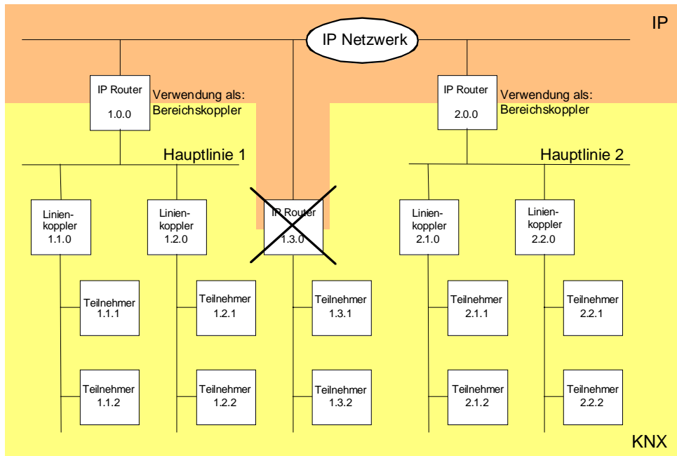
Bild 2: IP Router als Bereichskoppler
