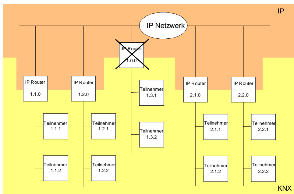
Bild 3: IP Router als Linienkoppler
