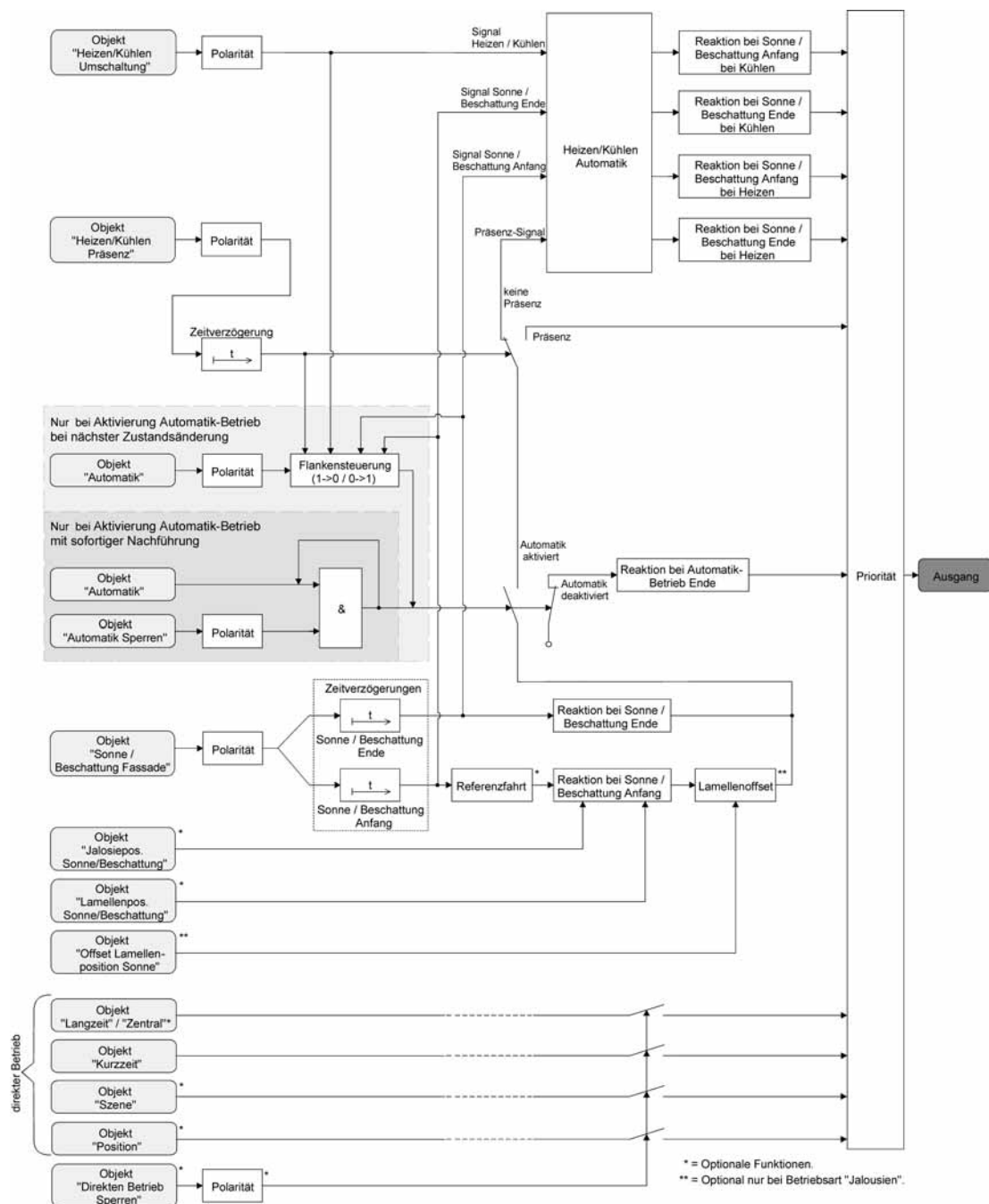
Bild 31: Funktionsschaltbild der Heizen/Kühlen-Automatik
