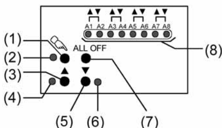
Bild 8: Bedien- und Anzeigeelemente der Handbedienung an der Gerätefront
