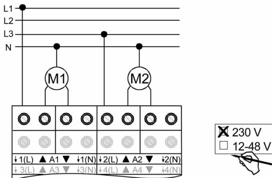
Bild 4: Elektrischer Anschluss für 230 V-Antriebsmotoren
