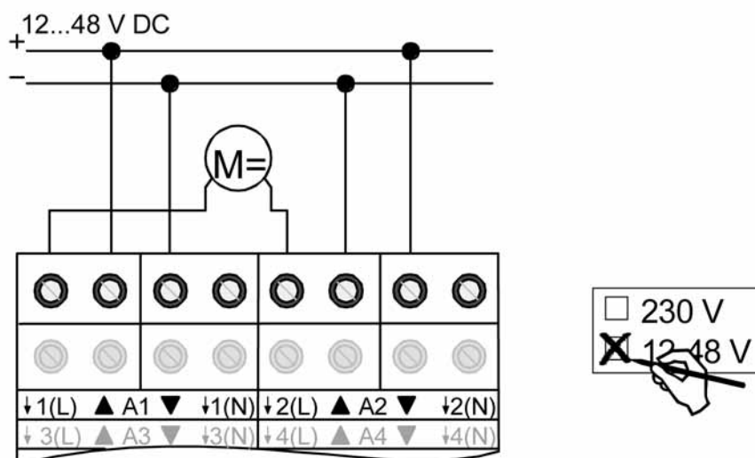
Bild 6: Elektrischer Anschluss für 12 ... 48 V-Antriebsmotoren
