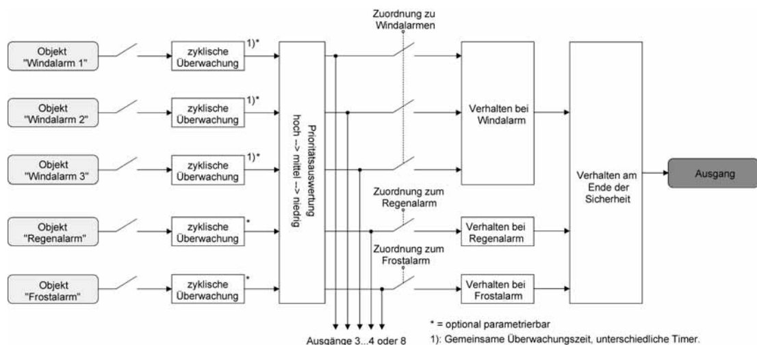
Bild 18: Funktionsschaltbild der kanalorientierten Sicherheitsfunktionen
