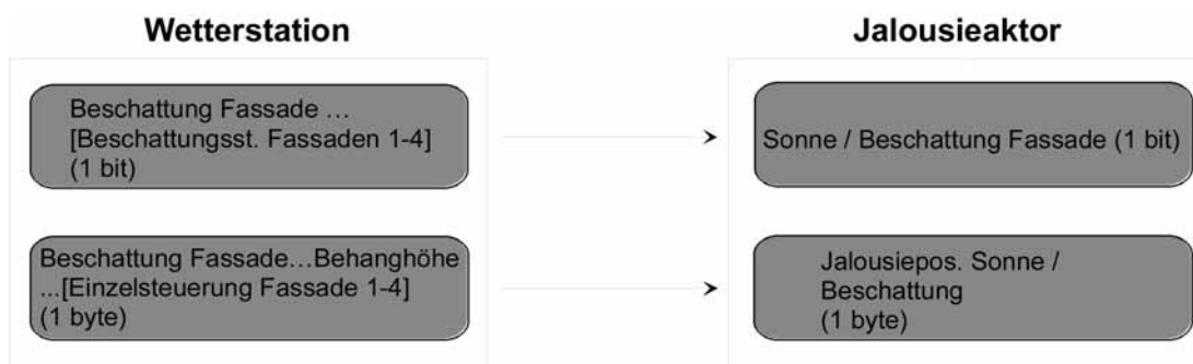
Bild 29: Projektierung der Kommunikationsobjekte für Anwendungsbeispiel V.
