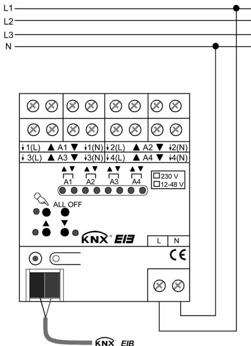
Bild 3: Elektrischer Anschluss der Netzspannungsversorgung
