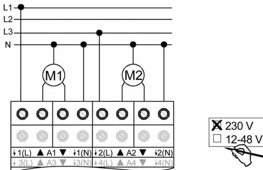
Bild 5: Elektrischer Anschluss für 230 V-Antriebsmotoren bei automatischer Endlagenerkennung
