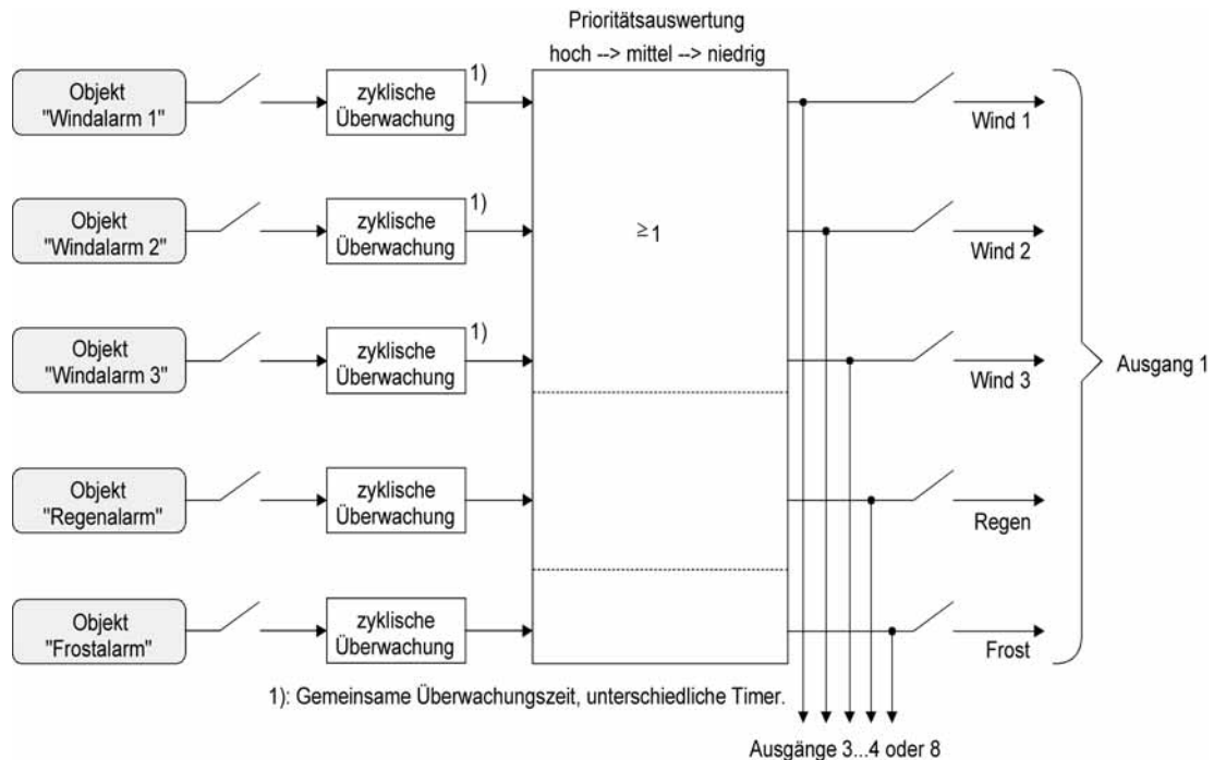
Bild 10: Funktionsschaltbild der Sicherheitsfunktionen
