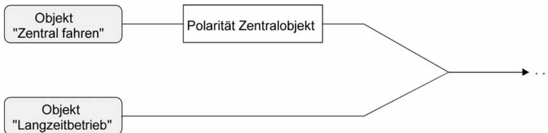
Bild 9: Funktionsschaltbild "Zentral fahren"
