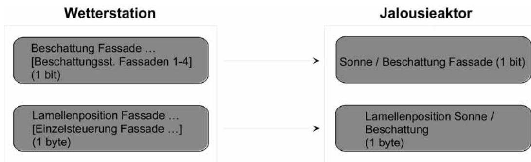
Bild 27: Projektierung der Kommunikationsobjekte für Anwendungsbeispiel III.
