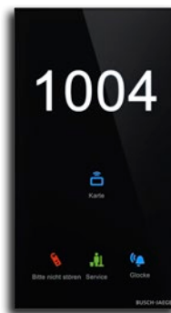
Raumaußensensor mit Kartenleser und Zimmernummer
