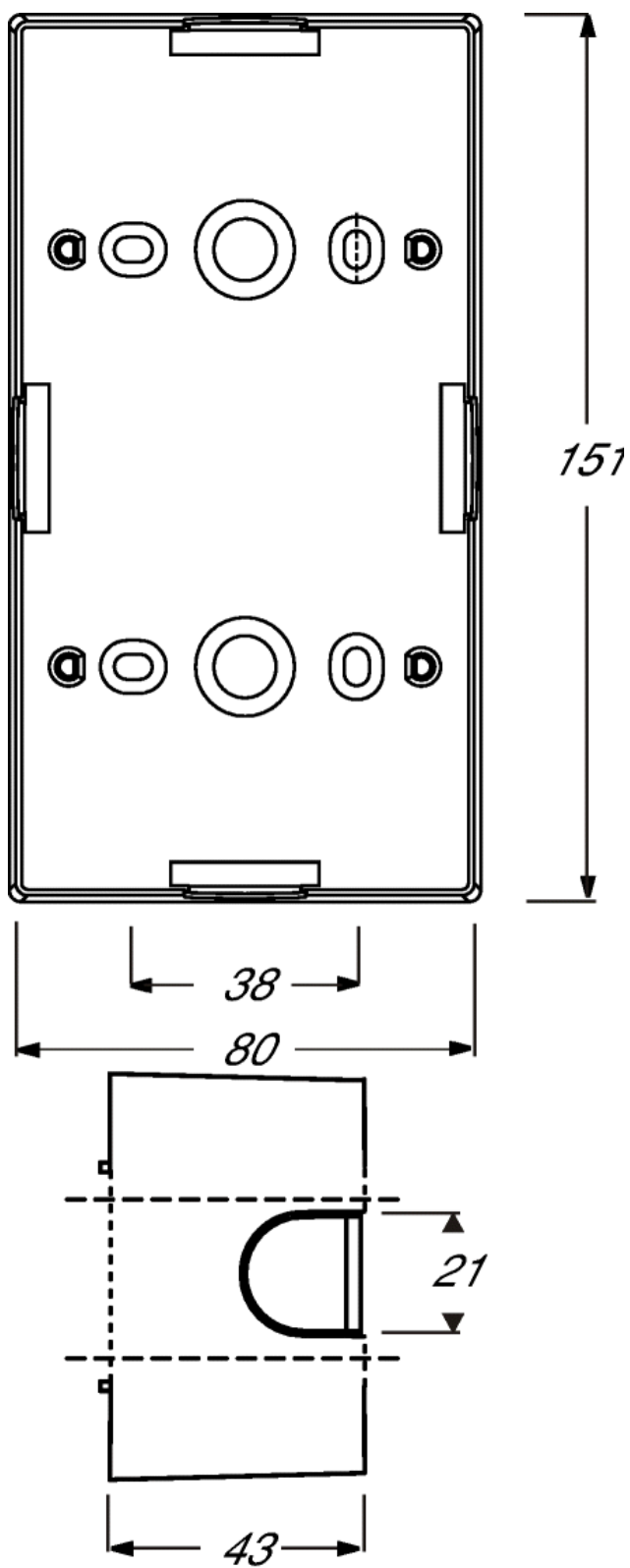
Aufputz-Gehäuse 2-fach für solo®, future® linear
