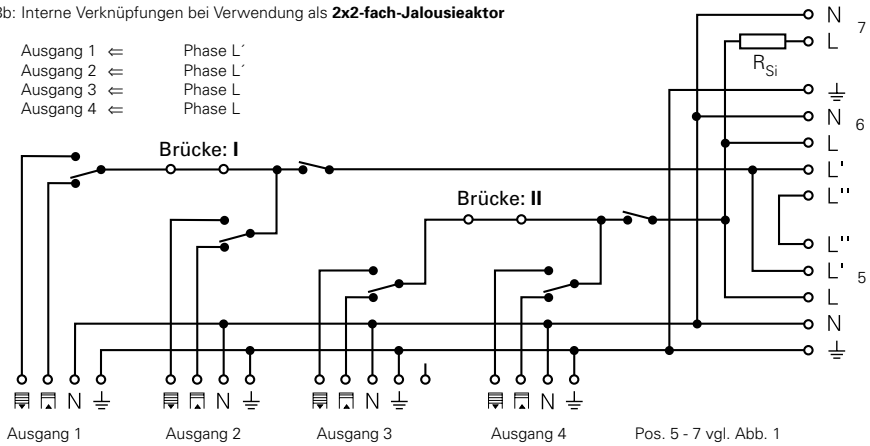
Abb. 3c: Interne Verknüpfungen bei Verwendung als kombinierter 2-fach-Schalt-/1x2-fach-Jalousieaktor
