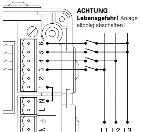
Abb. 6b: 230 V ~ (externer Mehrphasenbetrieb)
