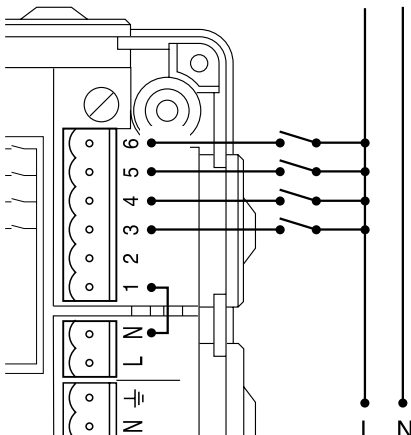
Abb. 6a: 230 V ~ (externer Einphasenbetrieb)
