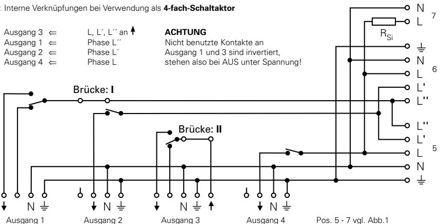
Abb. 3a: Interne Verknüpfungen bei Verwendung als 4-fach-Schaltaktor
