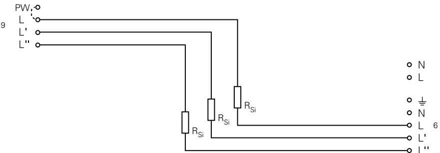
Abb. 3d: Interne Verknüpfung der Phasenwahl
