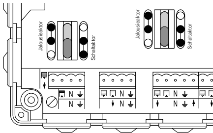
Abb. 2b: Lage und Stellung der Steckbrücken bei Betrieb als 2x2-fach-Jalousieaktor (Applikation V.3.1)
