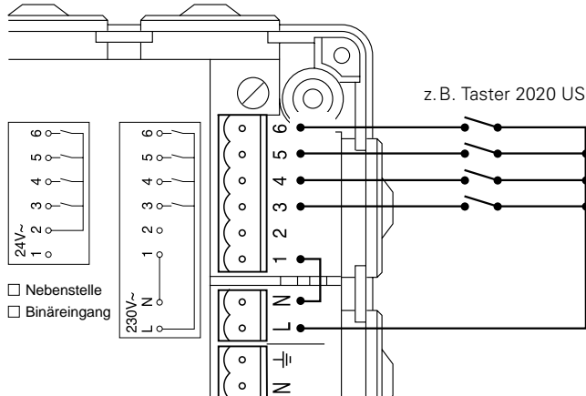
Abb. 5: 230 V ~ (intern)
