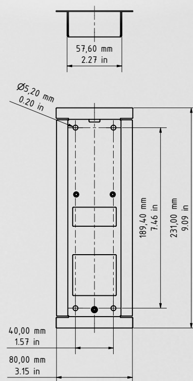
Montagerückgehäuse
