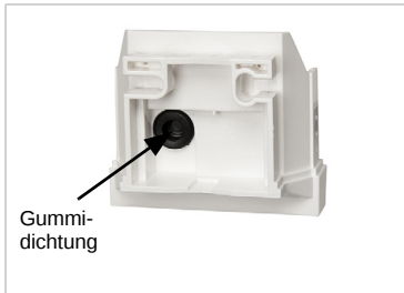
Abb. 8 Führen Sie das Anschlusskabel durch die Gummidichtung.
