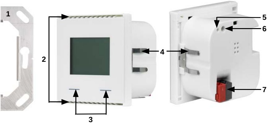
Abb. 2 1 Tragrahmen 2 Öffnungen für Luftzirkulation 3 Touch-Tasten 4 Rasten 5 Programmier-LED (versenkt) 6 Programmier-Taste (versenkt) zum Einlernen des Geräts
