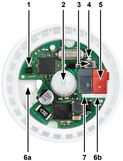
Abb. 4 1 Sensoren für Temperatur, Feuchtigkeit 2 Bewegungssensor 3 Programmier-Taster 4 Programmier-LED 5 KNX-Klemme BUS +/- 6 a+b Löcher für Befestigung (Lochabstand 30 mm) 7 Kabel-Durchführung (unter der KNX-Klemme)
