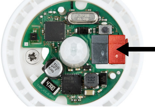
Abb. 8 Stecken Sie die KNX-Klemme mit dem Buskabel auf den Steckplatz.
