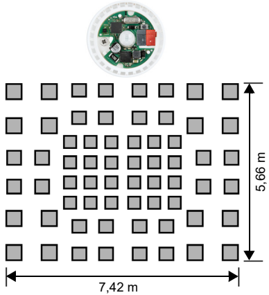
Abb. 1 Abstand 2,50 m
