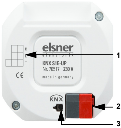
Abb. 3: Bus-Seite 1 Beschriftungsfeld 2 KNX-Steckklemme +/- 3 Programmier-LED und Programmier-Taste (versenkt)
