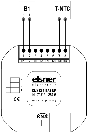
Beispiel KNX S1E-BA4-UP mit Binärkontakt an Eingang 1 und Temperatursensor T-NTC an Eingang 4.
