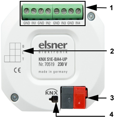
Abb. 2: Bus-Seite 1 Anschlussklemme Analog-/Digitaleingänge (nicht vorhanden bei KNX S1E-UP) 2 Beschriftungsfeld 3 KNX-Steckklemme +/- 4 Programmier-LED und Programmier-Taste (versenkt)
