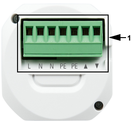
Abb. 1: Ausgangs-Seite 1 Anschluss-Klemme für Antrieb/Verbraucher 230 V AC
