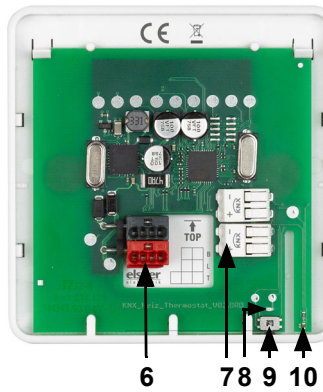
Abb. 3: Rückansicht ohne Halterung 6 KNX-Busklemme +/- für Anschluss bei Montage über einer Dose 7 Federkraftklemmen KNX-Bus für flächenbündige Montage direkt auf der Wand 8 Programmier-LED 9 Programmier-Taste (versenkt) zum Einlernen. 10 Temperatursensor
