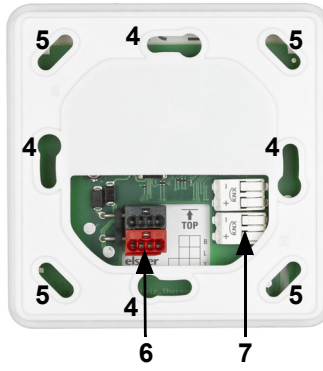
Abb. 2: Rückansicht mit Halterung 4/5 Schraublöcher für verschiedene Dosen. Die Befestigung mit 2 Schrauben ist ausreichend. Verwenden Sie bei Wandmontage ein für den Untergrund geeignetes Befestigungsmaterial! 6 KNX-Busklemme +/- für Anschluss bei Montage über einer Dose 7 Federkraftklemmen KNX-Bus für flächenbündige Montage direkt auf der Wand
