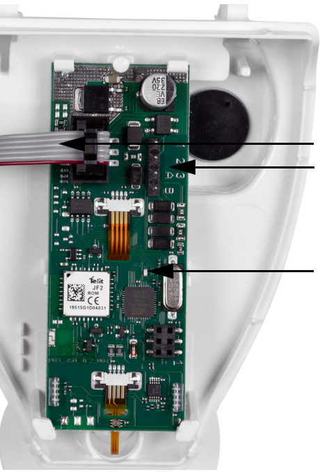
Abb. 12: Übersicht Platine 1 Kabelverbindung zum Nieder- schlagssensor im Gehäusede- ckel 2 Steckplatz für Anschlussstecker, geeignet für Massivleiter bis 0,8 mm² 1: +24 V DC | 2: GND A: Daten | B: Daten 3 Kontroll-LED GPS-Empfang
