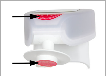
Abb. 15 Entfernen Sie nach der Montage den Schutz- aufkleber am Windsensor und den Hinweis- aufkleber „Abstand“ an der Oberseite des De- ckels.
