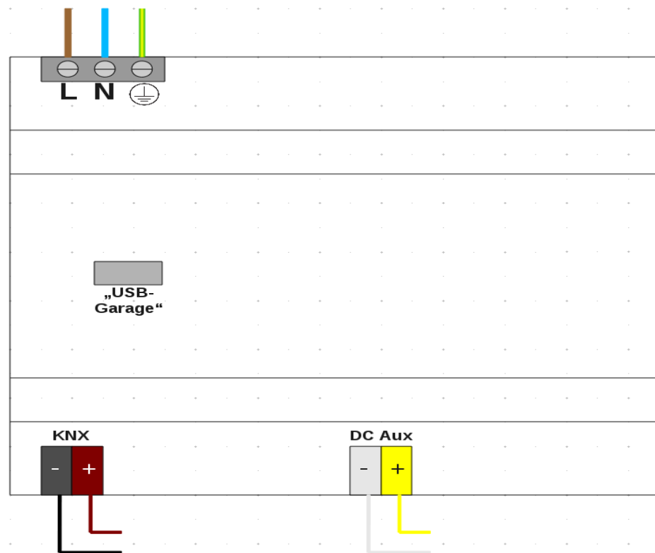
Abbildung 1: Anschlüsse
