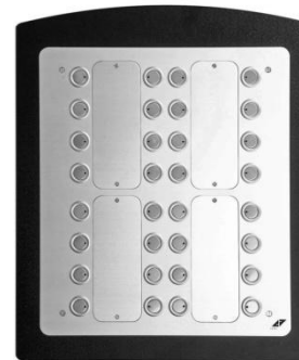
Aufputzgehäuse: 350 x 310 x 80 mm
