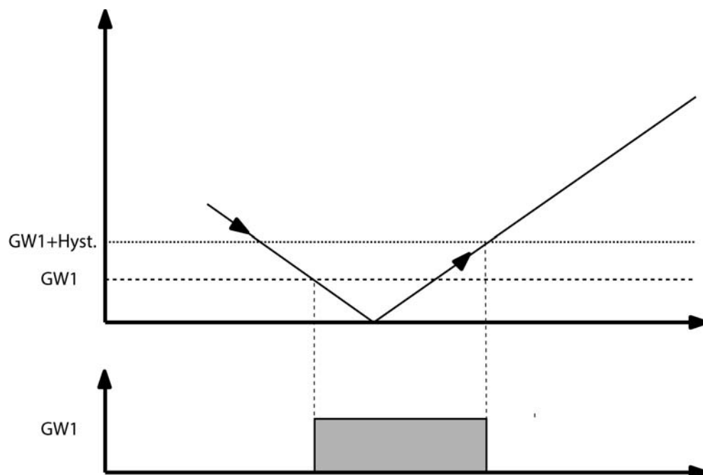
Bild 15: Aktivierung Grenzwert
