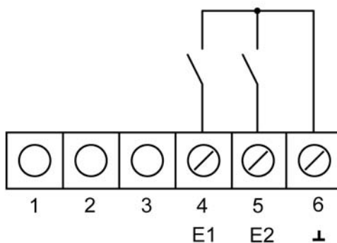
Bild 4: Anschluss Binäreingänge
