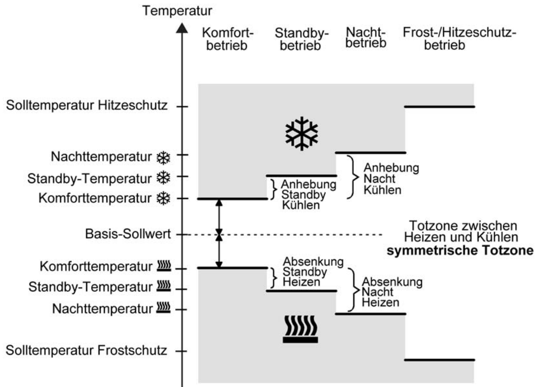
Bild 34: Solltemperaturen in der Betriebsart "Heizen und Kühlen" mit symmetrischer Totzone
