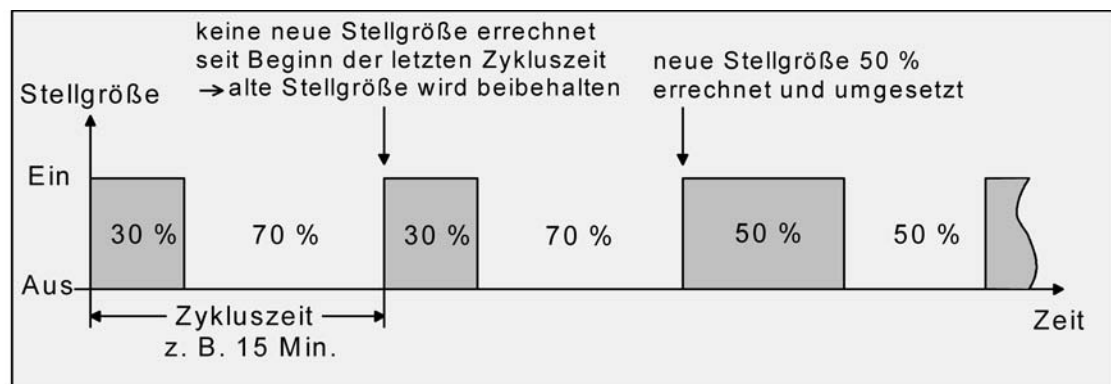
Bild 19: Schaltende PI-Regelung
