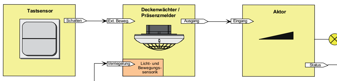
Bild 24: Applikationsbeispiel Einzelgerät mit externer Bewegungserfassung
