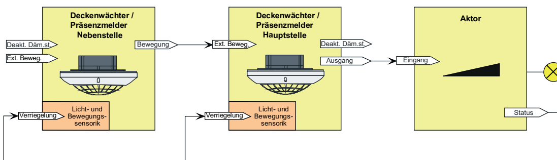
Bild 25: Applikationsbeispiel Haupt- und Nebenstelle ohne Dämmerungsstufenauswertung
