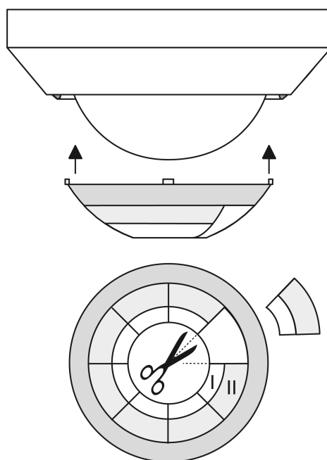
Bild 4: Einschränkung des Erfassungsbereichs durch Aufsteckblende
