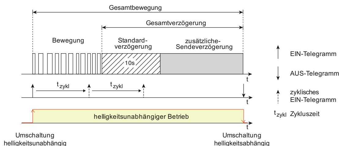
Bild 31: Gesamtbewegung mit Bewegungserfassung, Standardverzögerung und zusätzlicher Sendeverzögerung
