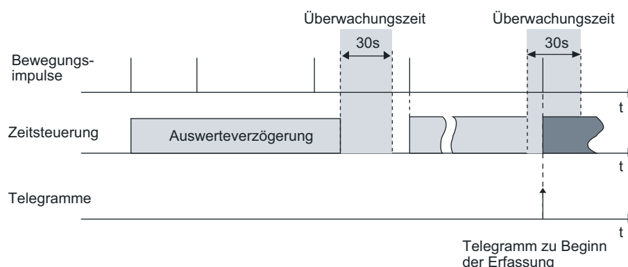
Bild 35: Auswerteverzögerung mit nur kurzzeitiger Bewegung
