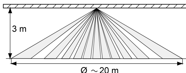
Bild 2: Durchmesser des Erfassungsbereichs bei Montagehöhe 3 m
