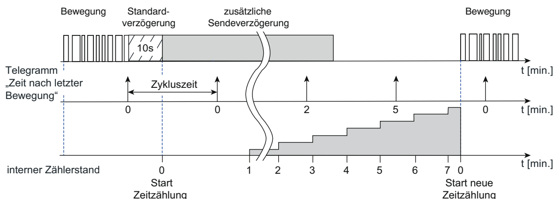
Bild 37: Messung der Zeitspanne nach letzter Bewegung
