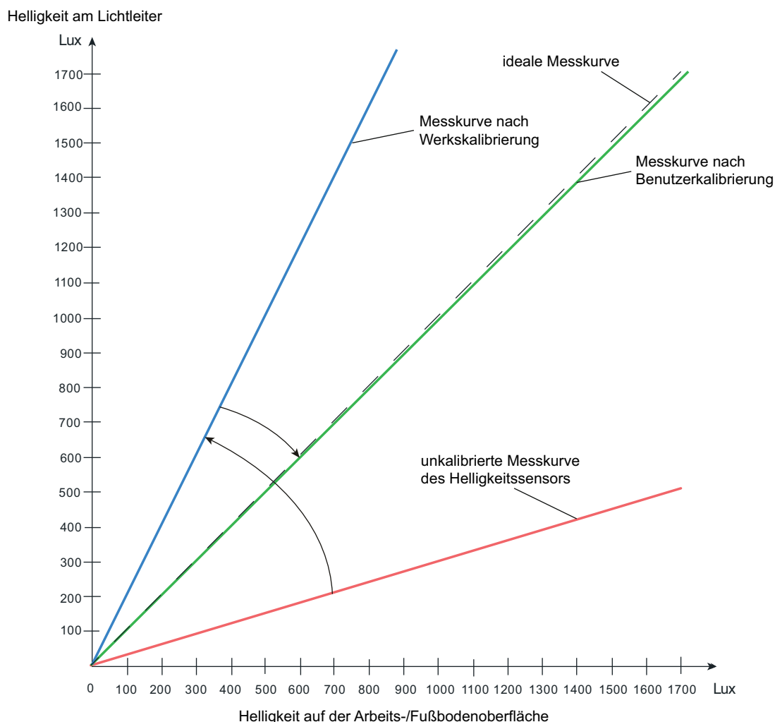
Bild 14: Korrektur der ermittelten Helligkeit an der Arbeits- / Fußbodenoberfläche durch Benutzerkalibrierung z. B. Reflexionsfaktor 0,5 entspricht Oberflächenbeschaffenheit (heller Fußbodenbelag)
