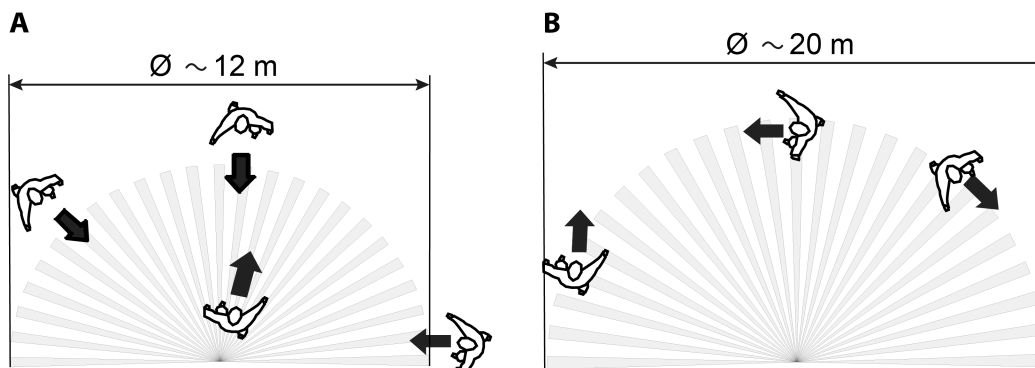
Bild 3: Erfassungsreichweite in Abhängigkeit der Bewegungsrichtung bei Montagehöhe 3 m
