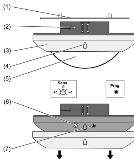
Bild 1: Geräteaufbau
