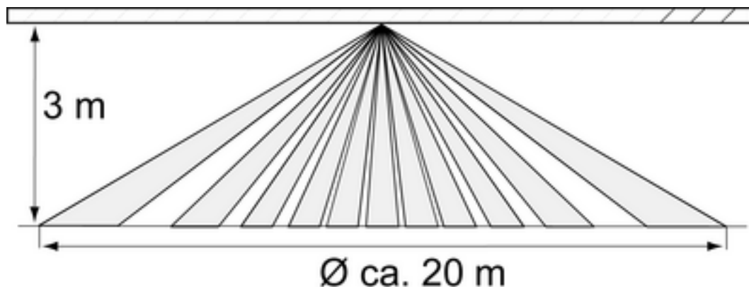
Bild 2: Sensorfenster und Erfassungsbereich
