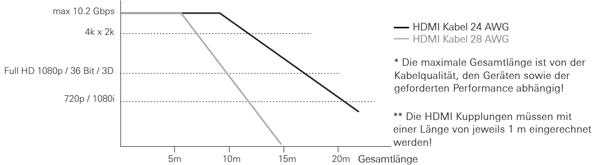
Performance in Abhängigkeit zur Gesamtlänge (vereinfachte Darstellung)
