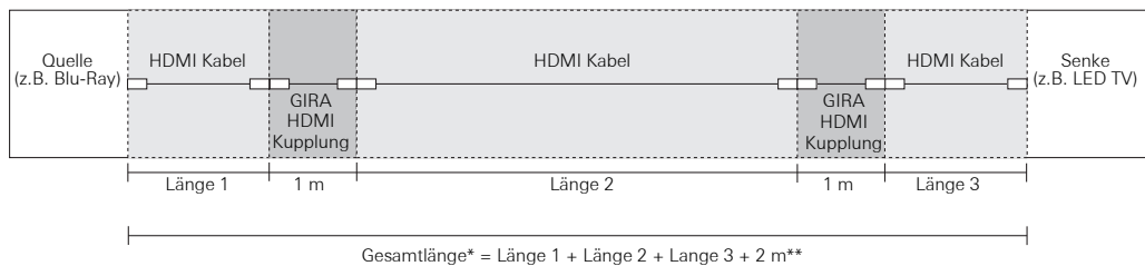
Performance in Abhängigkeit zur Gesamtlänge (vereinfachte Darstellung)
