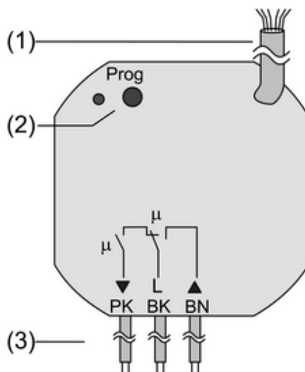
Bild 2: Jalousieaktor
