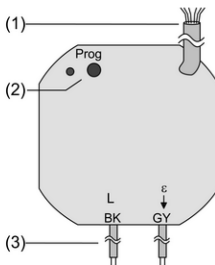
Bild 3: Heizungsaktor
