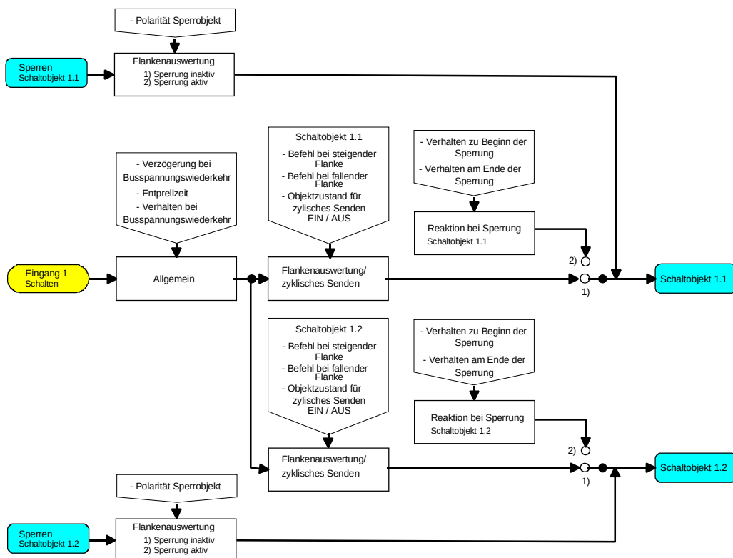
Funktionsschaltbild (für Binäreingang / z. B. Eingang 1 Funktion "Schalten")
