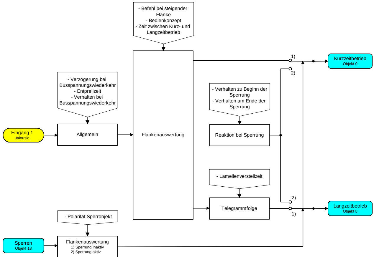
Funktionsschaltbild (für Binäreingang / z. B. Eingang 1 Funktion "Jalousie")
