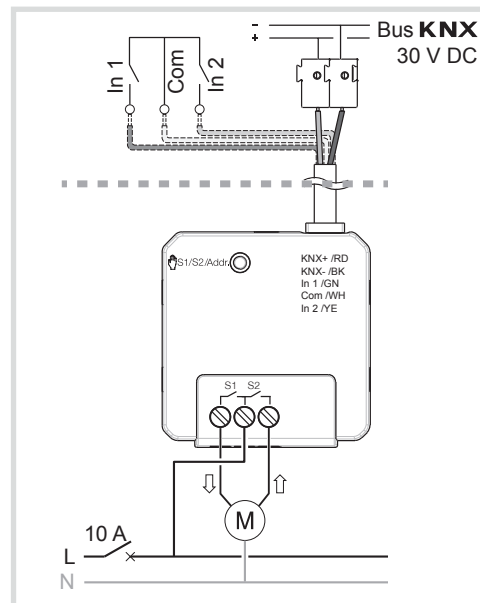
Bild 4: Anschluss von Motoren
