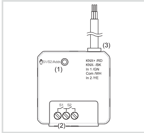
Figura 1: esempio di dispositivo con ingressi
