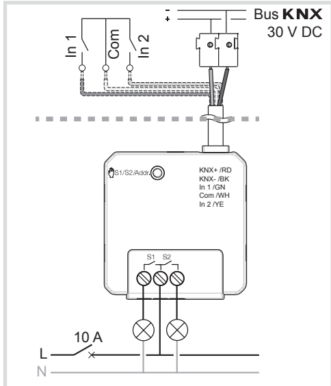
Figura 3: collegamento di carichi di commutazione
