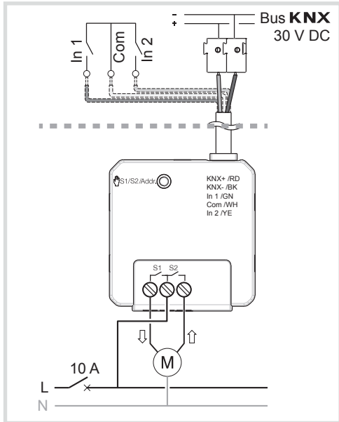
Figura 4: collegamento di motori
