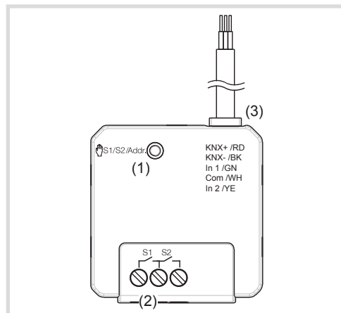
Bild 1: Beispiel Gerätevariante mit Eingängen
