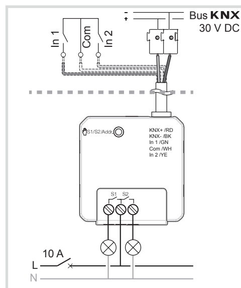
Bild 3: Anschluss von Schaltlasten
