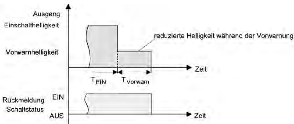
Bild 24: Die Vorwarnfunktion der Treppenhausfunktion ohne Soft-AUS-Funktion
