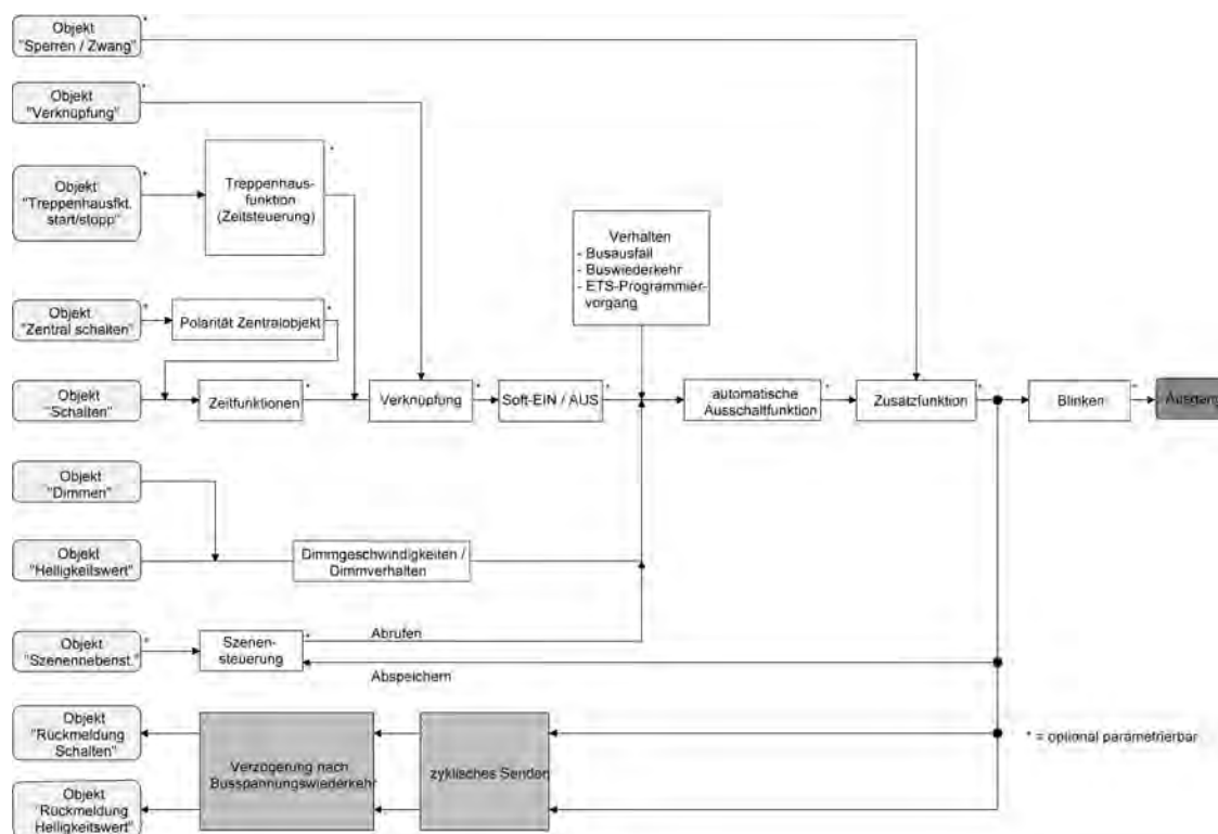
Bild 13: Funktionsschaltbild der Rückmeldungen
