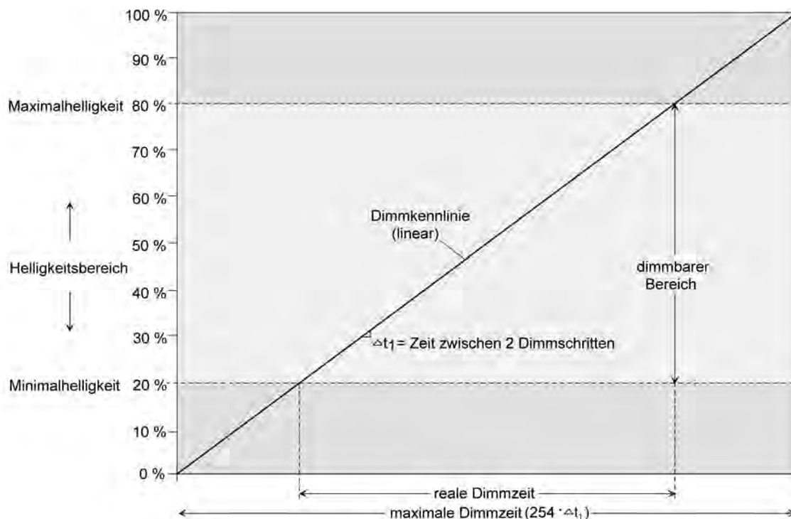
Bild 36: Lineare Dimmkennlinie als Beispiel mit Minimalhelligkeit > 0 % und Maximalhelligkeit
