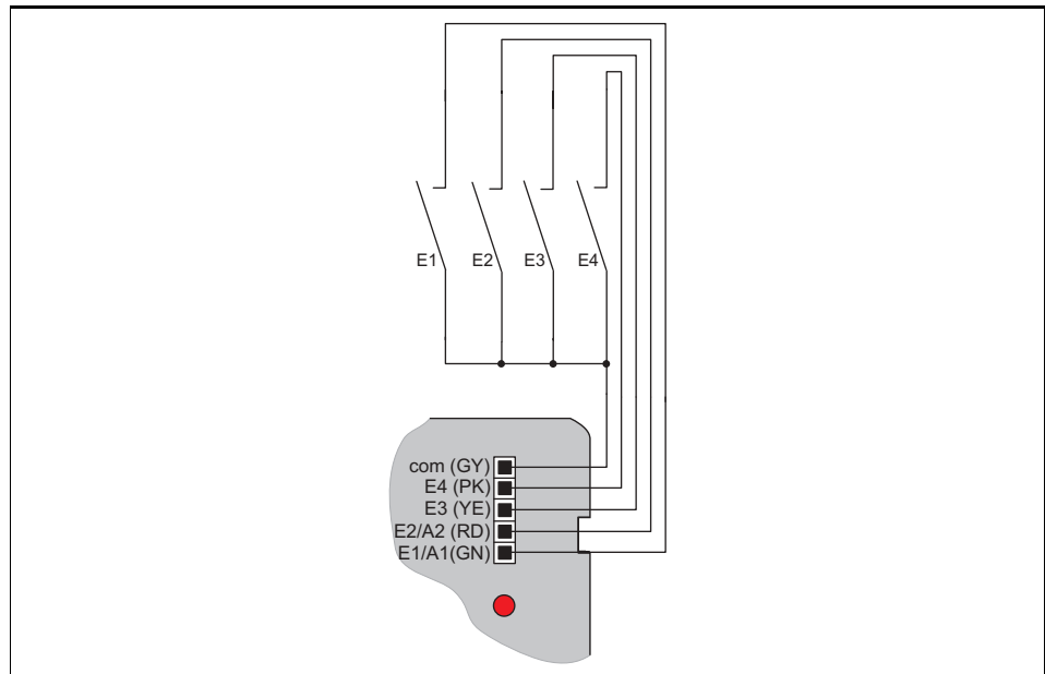
Bild 2: Beispiel Tasterschnittstelle 4fach mit 4 Eingängen
