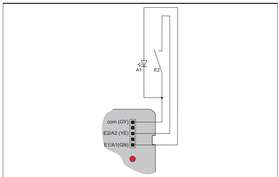
Bild 5: Beispiel Tasterschnittstelle 2fach verwendet mit 1 Eingang und 1 Ausgang
