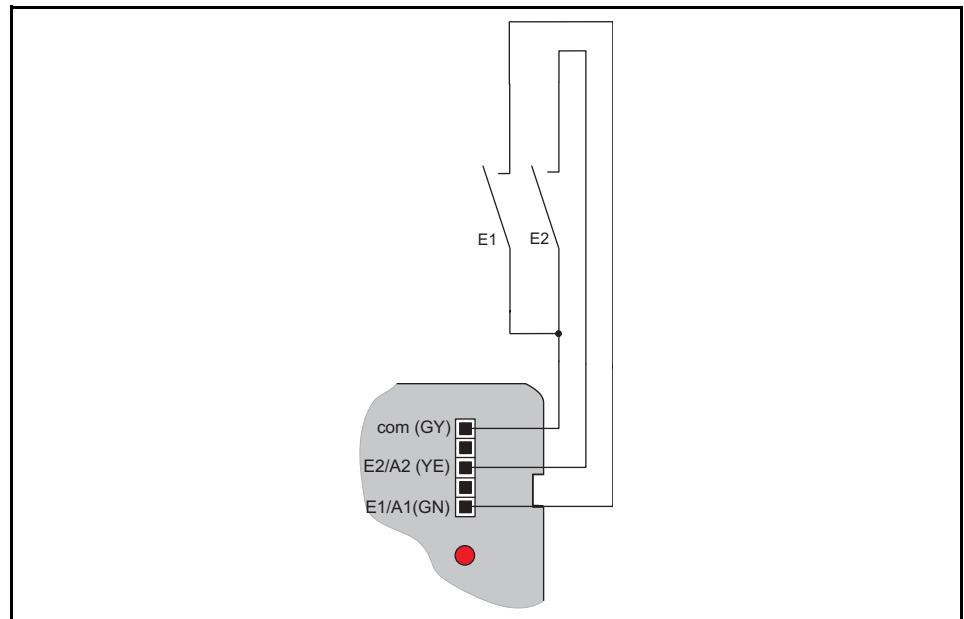
Bild 4: Beispiel Tasterschnittstelle 2fach mit 2 Eingängen
