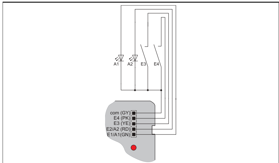
Bild 3: Beispiel Tasterschnittstelle 4fach verwendet mit 2 Eingängen und 2 Ausgängen
