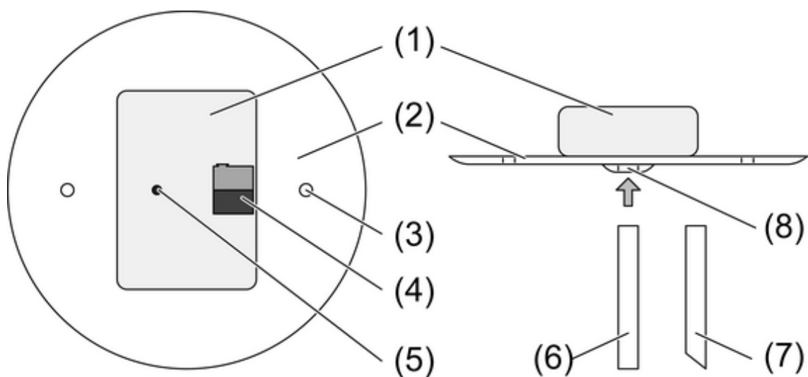
Bild 1: Helligkeitsregler Unterputz
