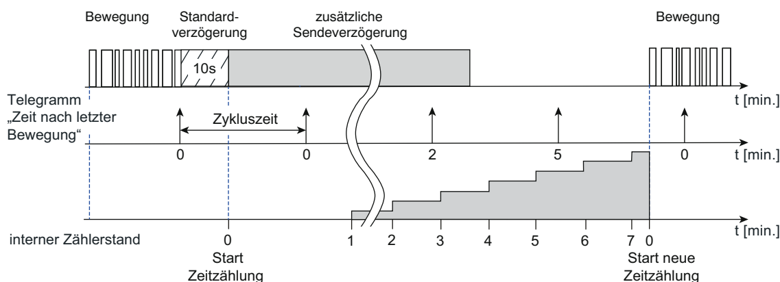
Bild 41: Messung der Zeitspanne nach letzter Bewegung
