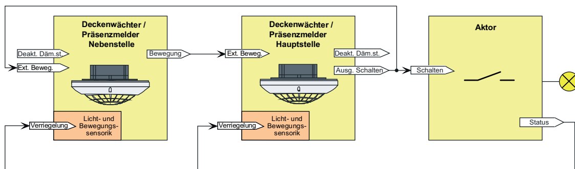
Bild 33: Applikationsbeispiel mit Dämmerungsstufenauswertung in der Hauptstelle und in den Nebenstellen für Ausgangsfunktion "Treppenhausfunktion"
