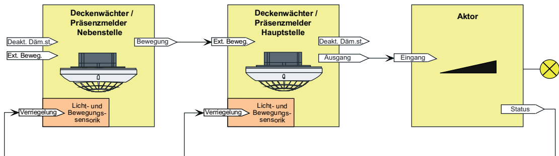
Bild 30: Applikationsbeispiel Haupt- und Nebenstelle mit Dämmerungsstufenauswertung in der Hauptstelle
