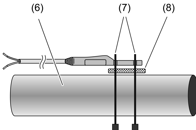
Bild 2: Montage mit Kabelbindern auf Rohrleitung
