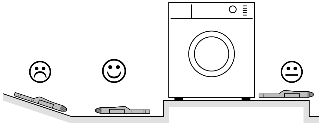
Bild 3: Geeignete und ungeeignete Montageorte
