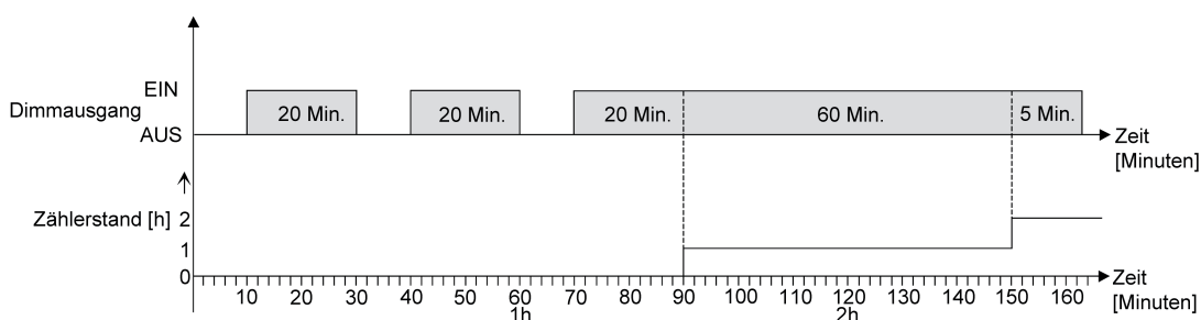
Bild 37: Funktionsweise des Betriebsstundenzählers (am Beispiel eines Vorwärtzählers)
