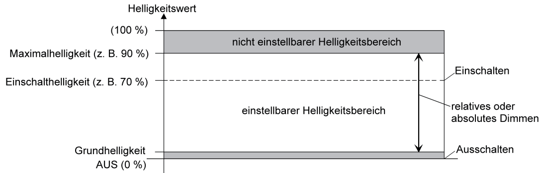
Bild 11: Beispiel eines Helligkeitsbereichs mit Grundhelligkeit
