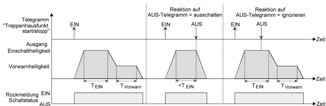
Bild 24: Ausschaltverhalten der Treppenhausfunktion mit Soft-Funktionen (als Beispiel mit Minimalhelligkeit = 0 %)
