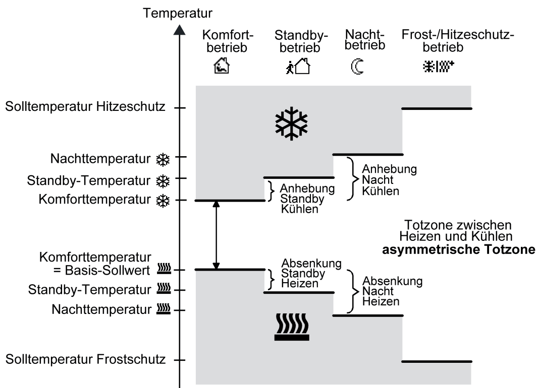
Bild 48: Solltemperaturen in der Betriebsart "Heizen und Kühlen" mit asymmetrischer Totzone
