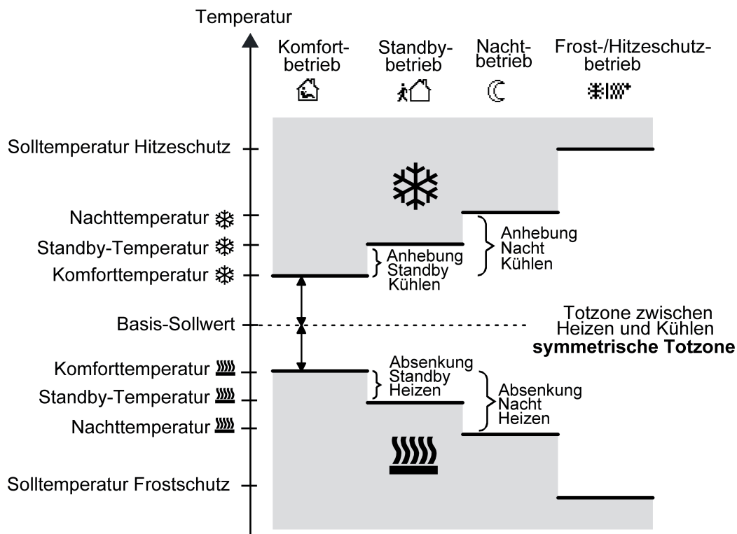
Bild 47: Solltemperaturen in der Betriebsart "Heizen und Kühlen" mit symmetrischer Totzone
