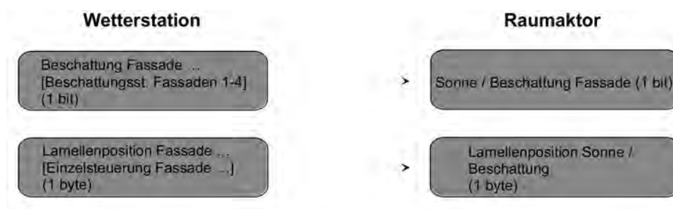
Bild 45: Projektierung der Kommunikationsobjekte für Anwendungsbeispiel III.
