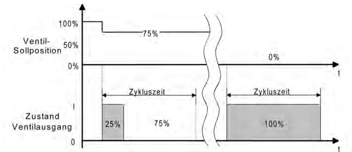
Bild 54: Umsetzung einer stetigen Ventil-Sollposition in ein Ausgangssignal bei stromlos geöffneten Ventilantrieben (Beispiel)
