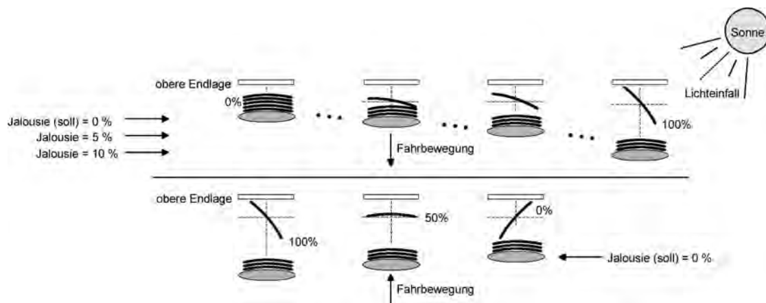
Bild 34: Beispiel für Lamellenpositionierung bei Jalousieposition in der oberen Endlage (Beispielhaft für Lamellentyp 1.)
