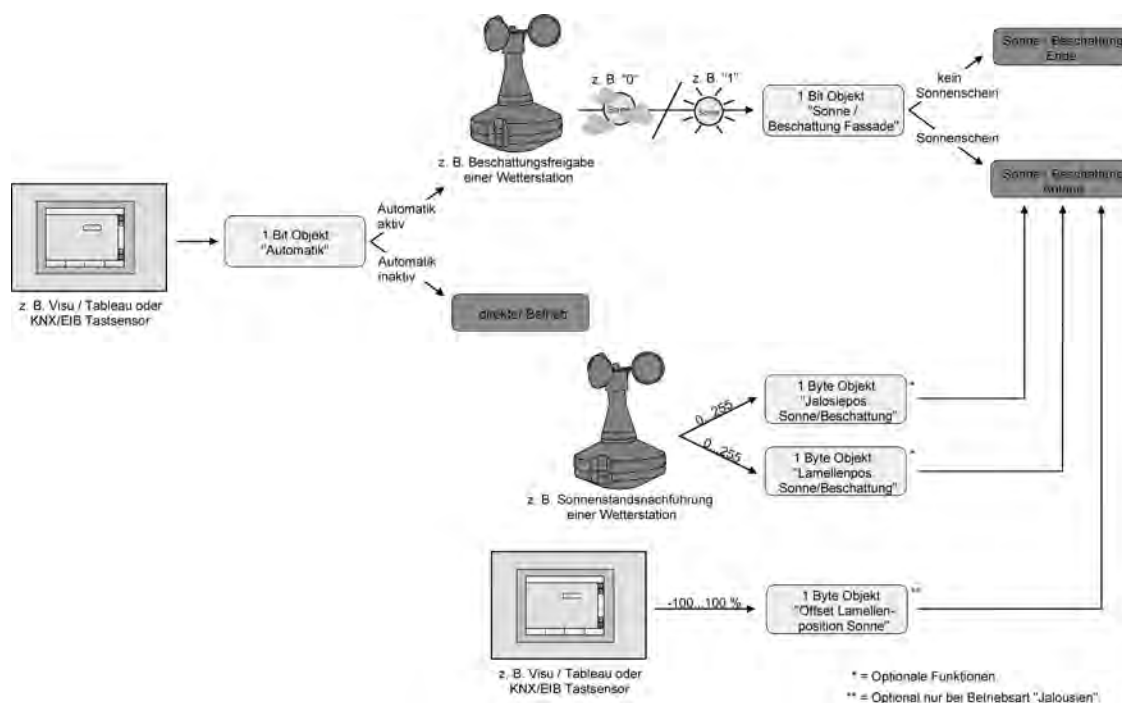
Bild 40: Prinzipschaltbild des erweiterten Sonnenschutzes (zur Vereinfachung ohne Sperrfunktionen)
