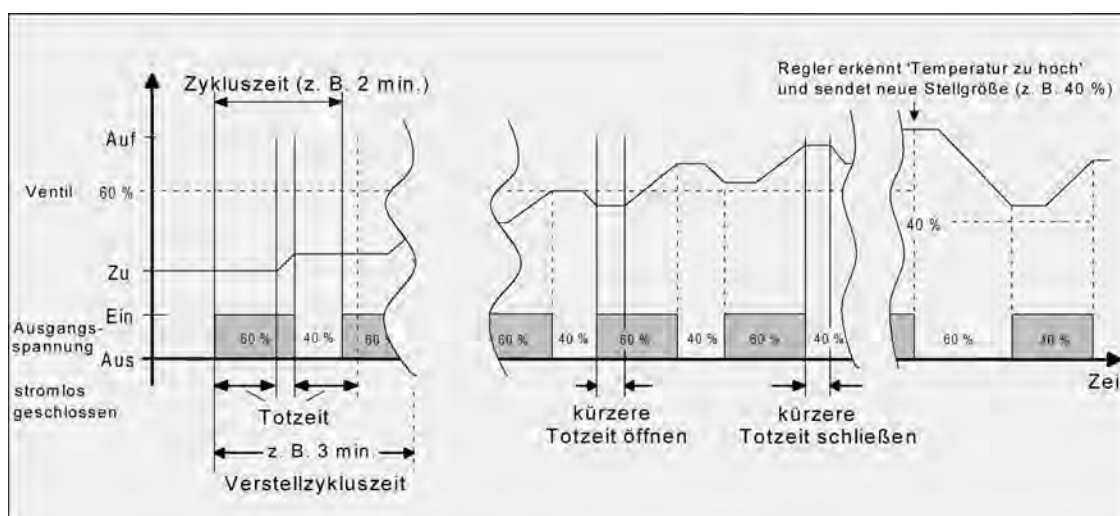
Bild 66: Idealisierter Verlauf des Ventilhubes exemplarisch dargestellt für eine Stellgröße von zunächst ca. 60 % eines stromlos geschlossenen Ventils
