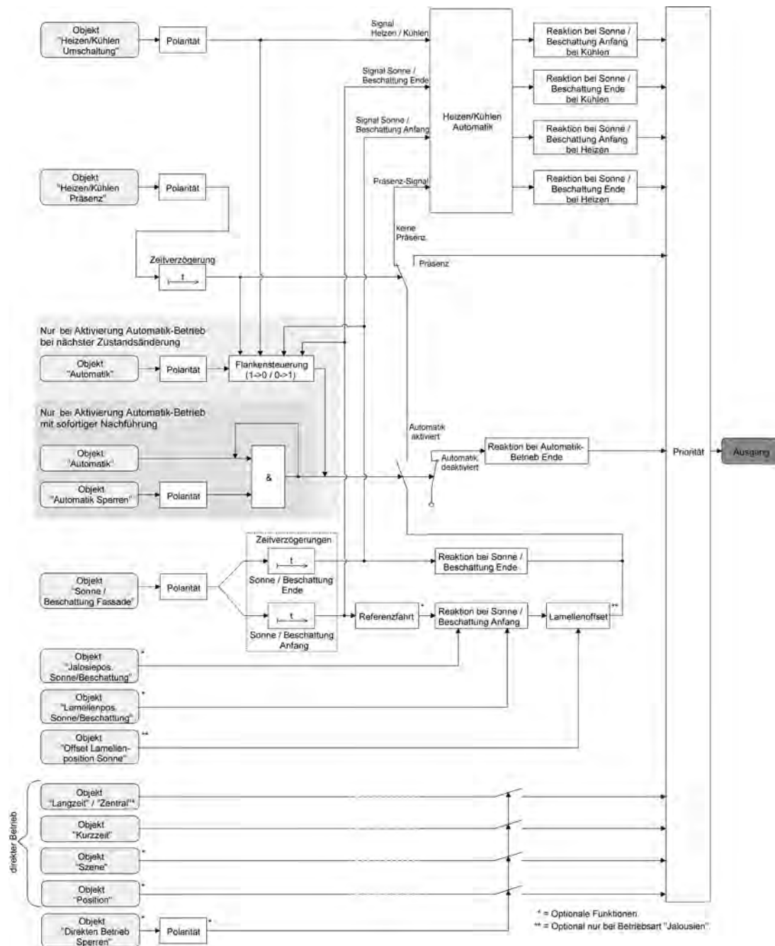
Bild 49: Funktionsschaltbild der Heizen/Kühlen-Automatik
