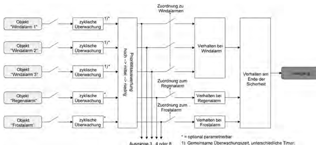
Bild 36: Funktionsschaltbild der kanalorientierten Sicherheitsfunktionen
