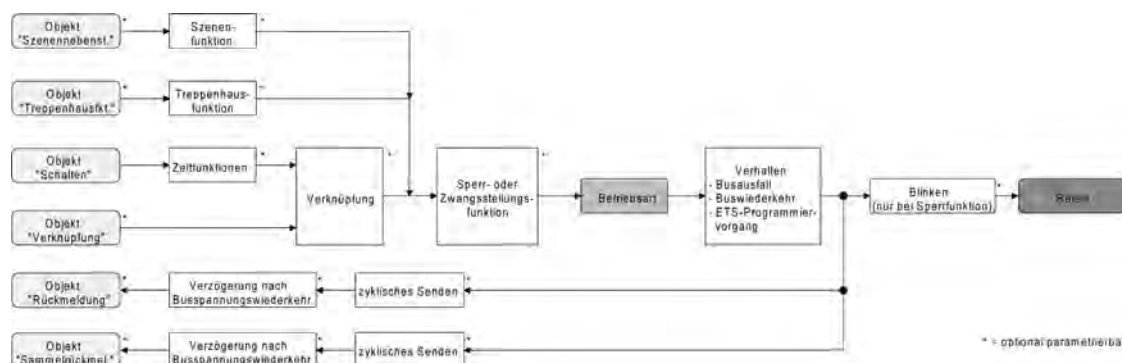
Bild 14: Funktionsschaltbild "Betriebsart"
