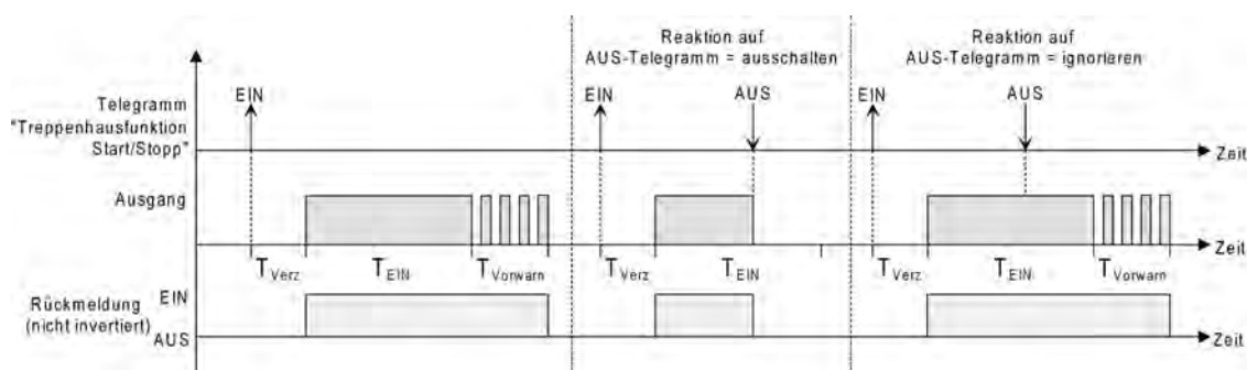
Bild 19: Ausschaltverhalten der Treppenhausefunktion
