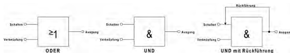
Bild 27: Verknüpfungsarten der Verknüpfungsfunktion
