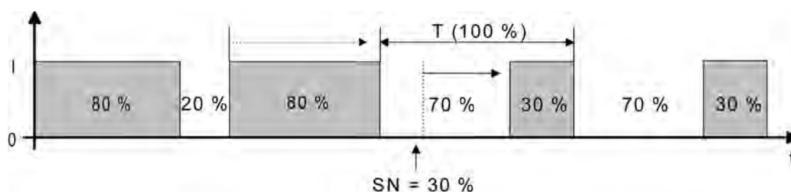
Bild 60: Stellgrößenänderung z. B. von 80 % auf 30 % während Schließphase des Ventils
