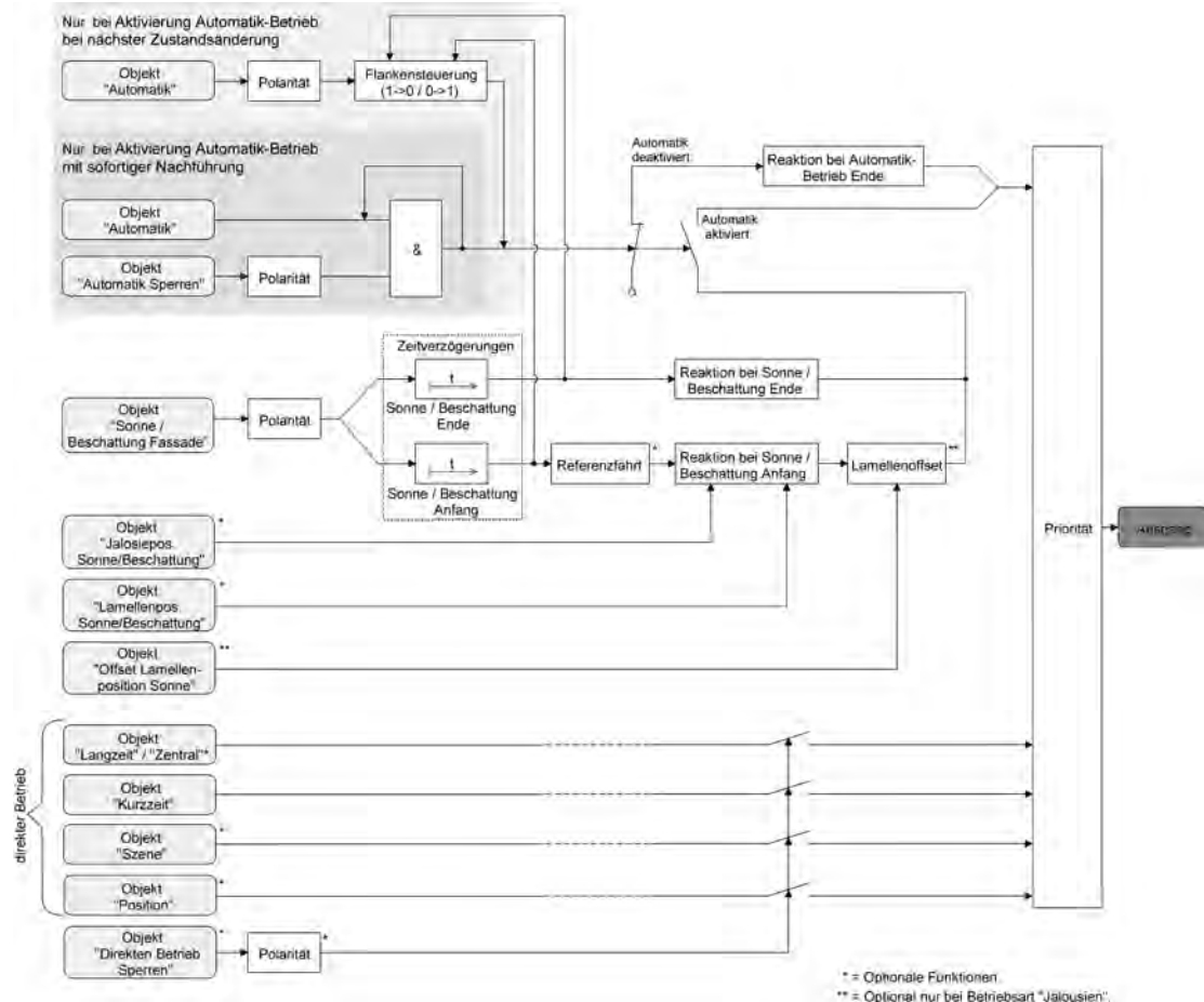
Bild 41: Funktionsschaltbild des erweiterten Sonnenschutzes
