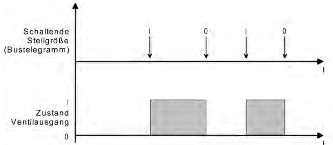
Bild 51: Umsetzung einer schaltenden Stellgröße in ein Ausgangssignal bei stromlos geschlossenen Ventilantrieben (Beispiel)
