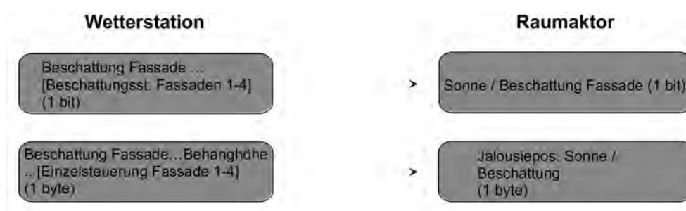
Bild 47: Projektierung der Kommunikationsobjekte für Anwendungsbeispiel V.
