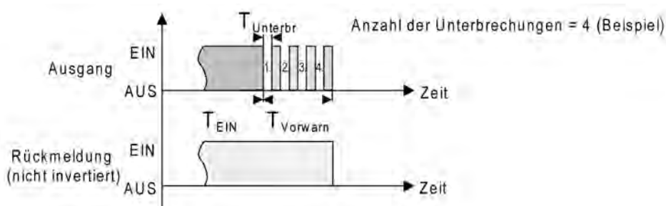
Bild 20: Die Vorwarnfunktion der Treppenhausfunktion (Beispiel)
