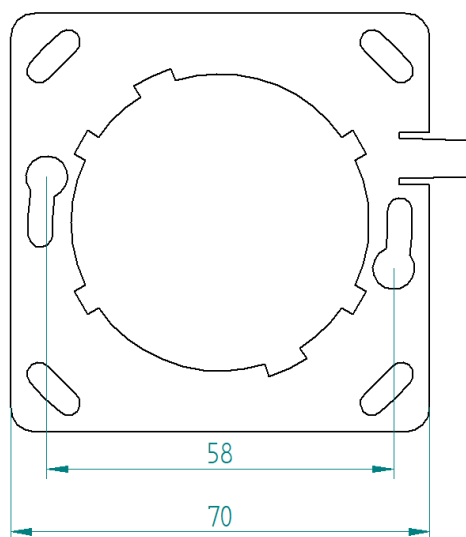
Abb. 2 Montageplatte
