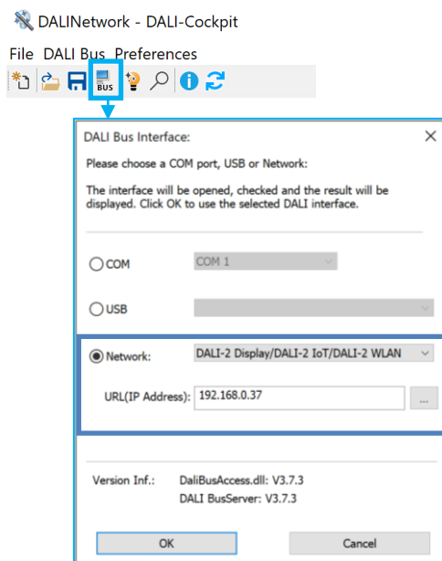
Abb. 14 DALI Cockpit –DALI Bus Schnittstelle
