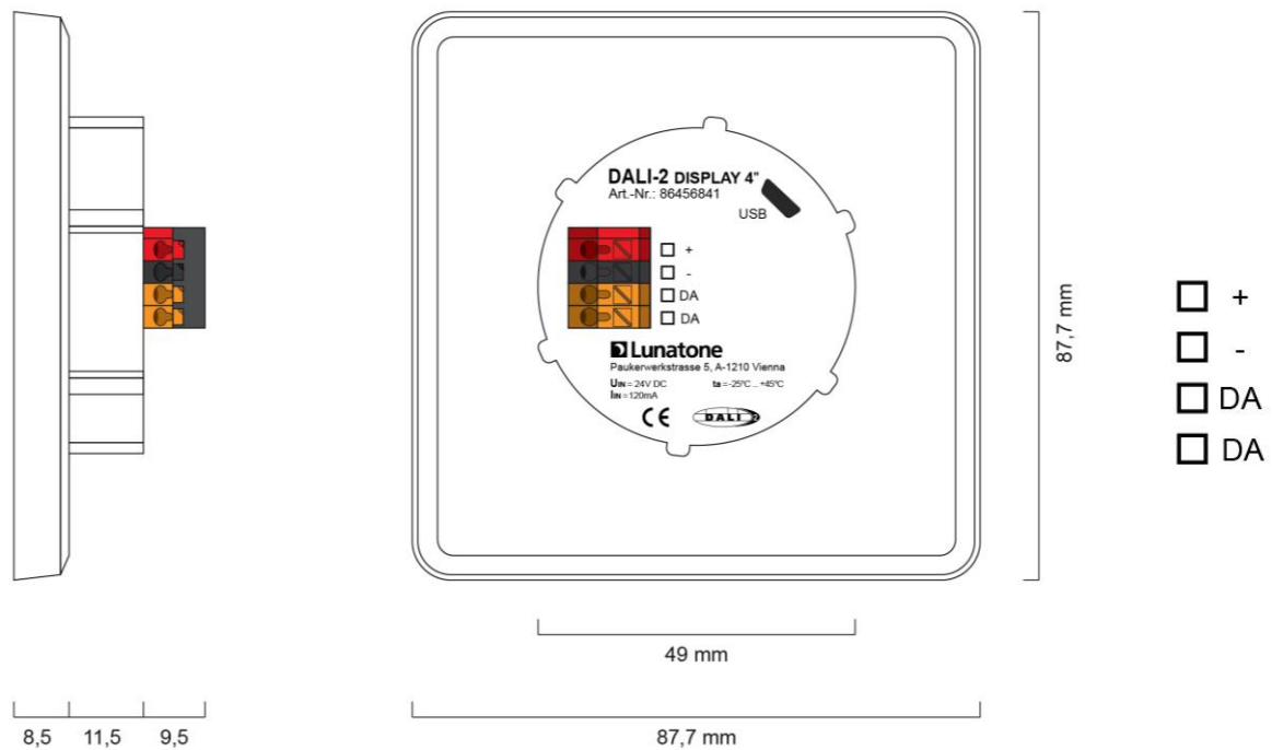
Abmessungen Art.Nr.: 86456841-...
