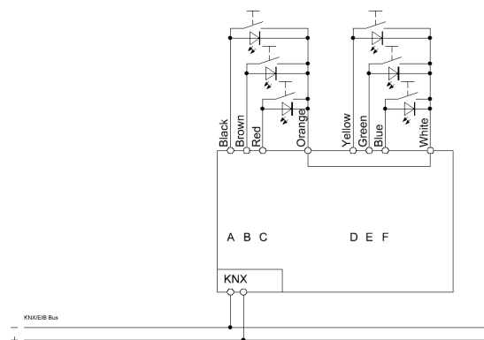
Anschlussbeispiel BE-06001.01
