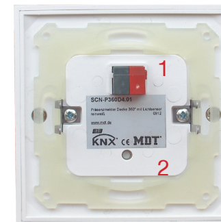
SCN-P360x4.02 Rückansicht - Back view
