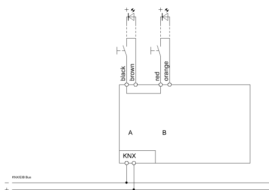
Anschlussbeispiel BE-02001.01
