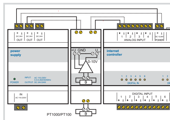
Anschlussbild Spannungsmessung 0-10V
