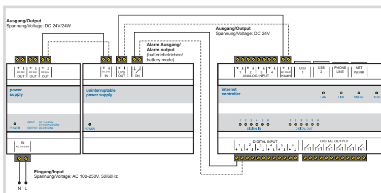
Anschluss mit Spannungsversorgung DC 24V REG-K und USV Erweiterungsmodul REG-K
