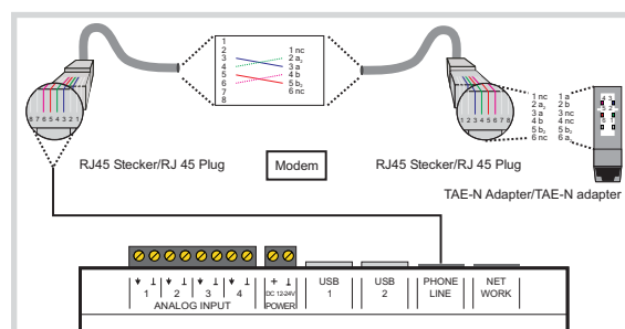
Anschlussbild analoger Telefonanschluss
