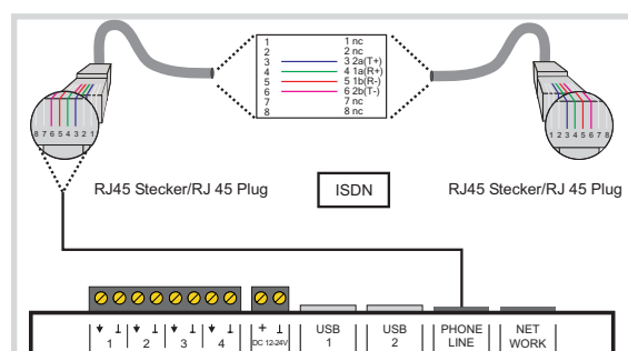
Anschlussbild ISDN Telefonanschluss
