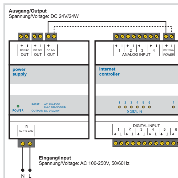
Anschluss mit Spannungsversorgung DC 24V REG-K
