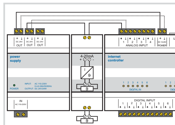
Anschlussbild Strommessung 0-20mA
