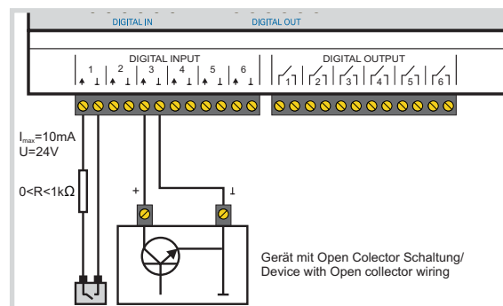
Anschlussbild digitale Eingänge
