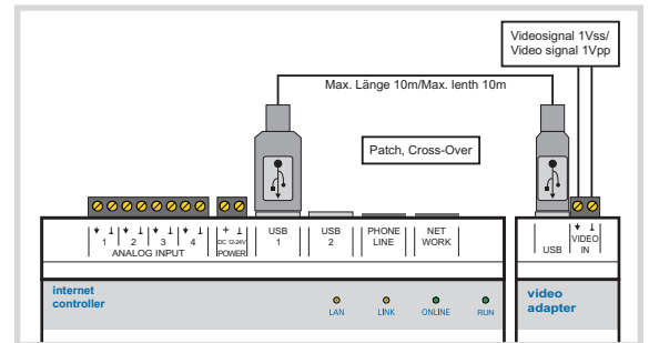
Anschlussbild USB-Geräteanschluss mit USB Video Adapter REG-K
