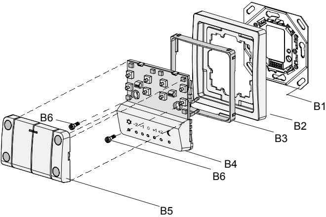
Bild 1: Montage des Raumtemperaturregler UP 231/3
