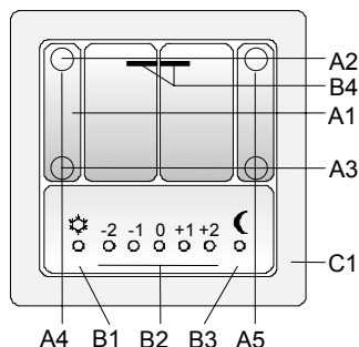
Bild 2: Lage der Anzeige- und Bedienelemente
