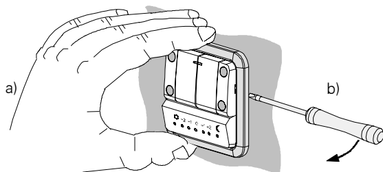
Bild 5: Demontage
