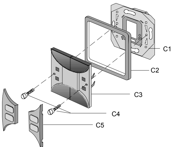
Bild 2: Montage des Tasters (Prinzipdarstellung)
