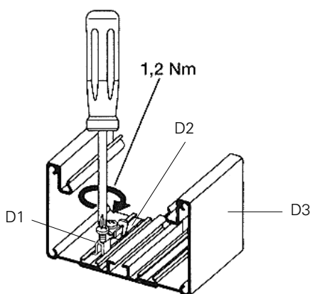
Bild 4: Fixierung der Erdungsklemmen Vor der Montage der Module (E1) im Kanal wird auf den Flachsteckeranschluß (E2) am Modul der Kabelschuh der Schutzleiterlitze (E3) aufgesteckt. Über die Schutzleiterlitze wird die Erdverbindung zur im Kanalunterteil montierten Erdungsklemme (E4) erzeugt.
