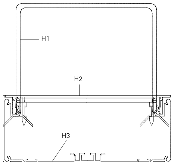
Bild 10: Position der Demontagehaken im Profilquerschnitt
