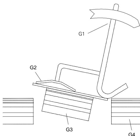
Bild 8: Hebelrichtung bei der Demontage
