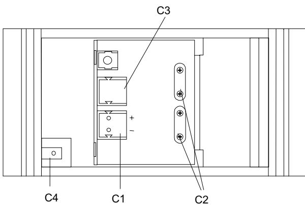
Bild 3: Rückseitige Modulansicht bei geöffnetem Deckel
