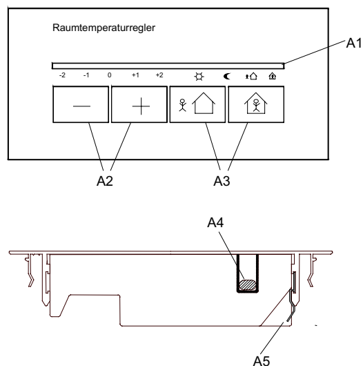
Bild 1: Lage der Anzeige- und Bedienelemente
