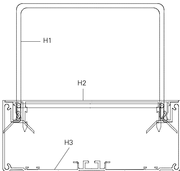
Bild 10: Position der Demontagehaken im Profilquerschnitt
