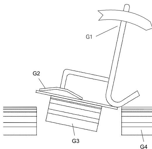
Bild 8: Hebelrichtung bei der Demontage
