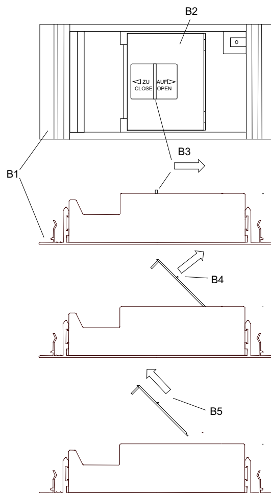
Bild 2: Öffnen des Gehäusedeckels
