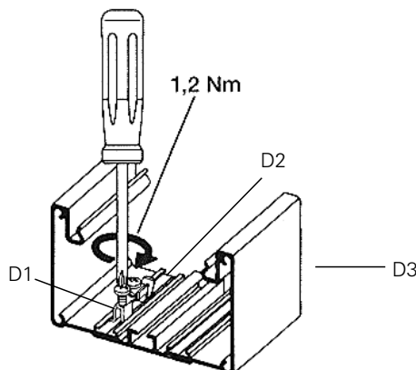
Bild 4: Fixierung der Erdungsklemmen
