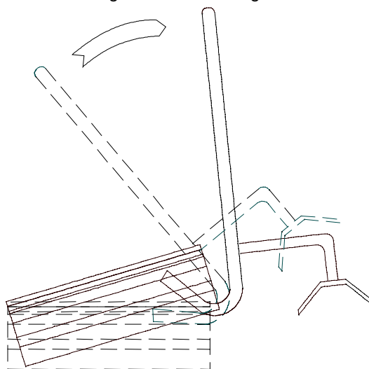
Bild 11: Heraushebeln des Kanaloberteils bzw. der Module
