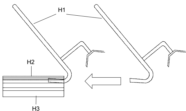
Bild 9: Ansetzen des Demontagewerkzeuges, um Kanaloberteile zu demontieren (Seitenansicht)
