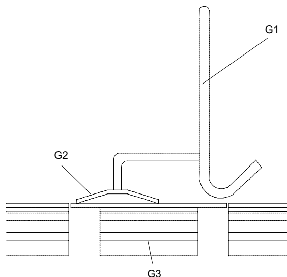
Bild 7: Aufsetzen des Demontagewerkzeugs
