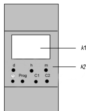
Bild 3: Lage der Anzeige- und Bedienelemente
